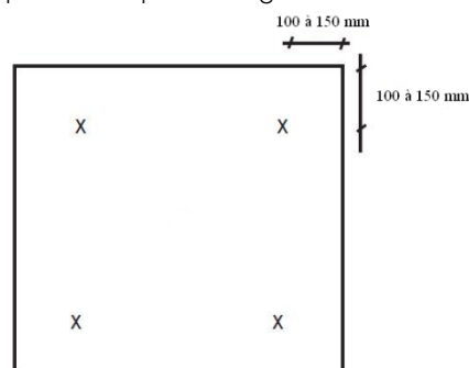
Fig. 1 – Schémas de pose pour les fixations mécaniques
