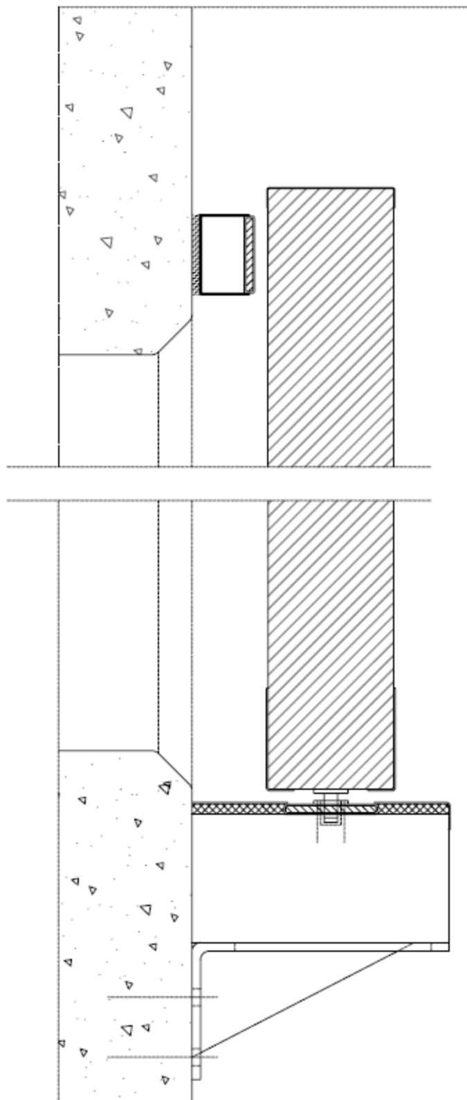
Figure 8 b : Serrure à crochet Coupe horizontale
