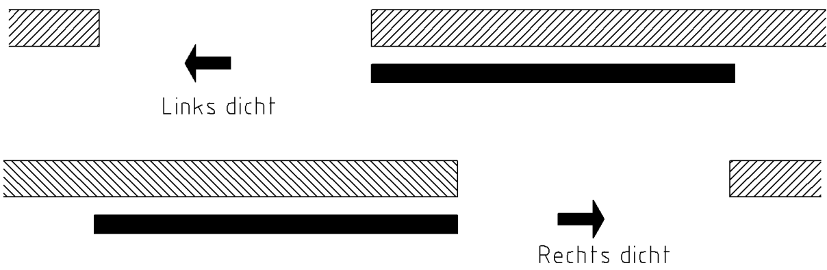
Figuur 2 : Schuifrichting
