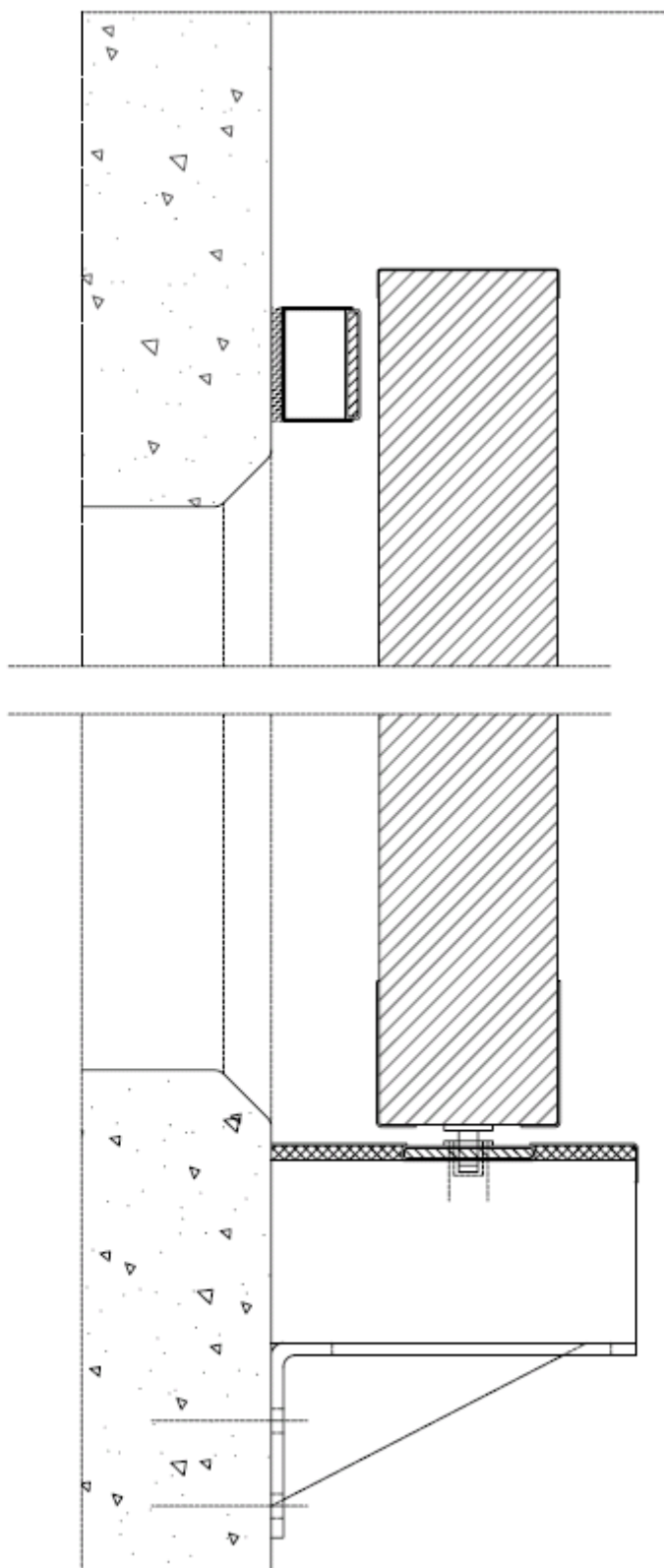
Figuur 8b : Haakslot Horizontale doorsnede
