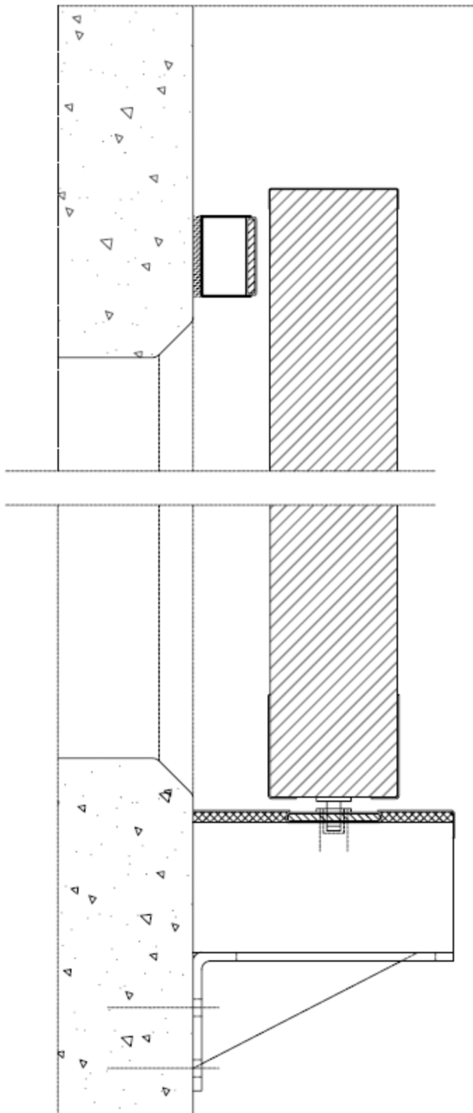
Figure 8b : Serrure à crochet Section horizontale
