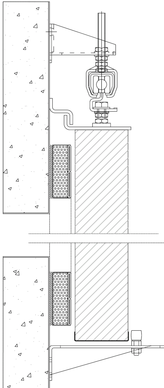
Figuur 5d : Omlijsting Vertikale doorsnede
