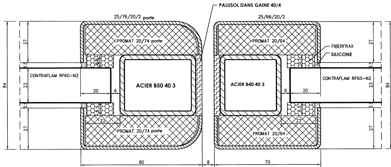
Coupes 5 et 7 : Raccord vantail-panneau latéral (côté latéral)
