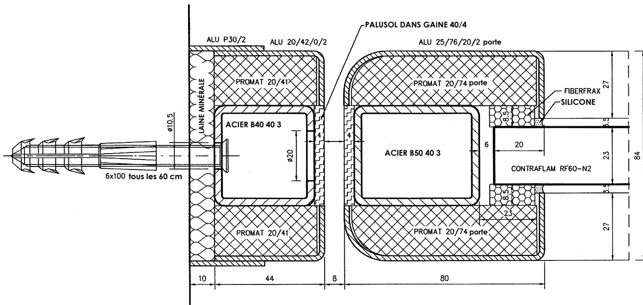
Coupes 1 et 2 : Raccords vantail-mur (côté latéral)
