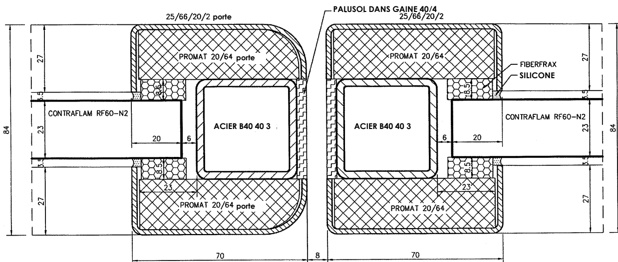
Coupes 5 et 7 : Raccord vantail-panneau latéral (côté latéral)
