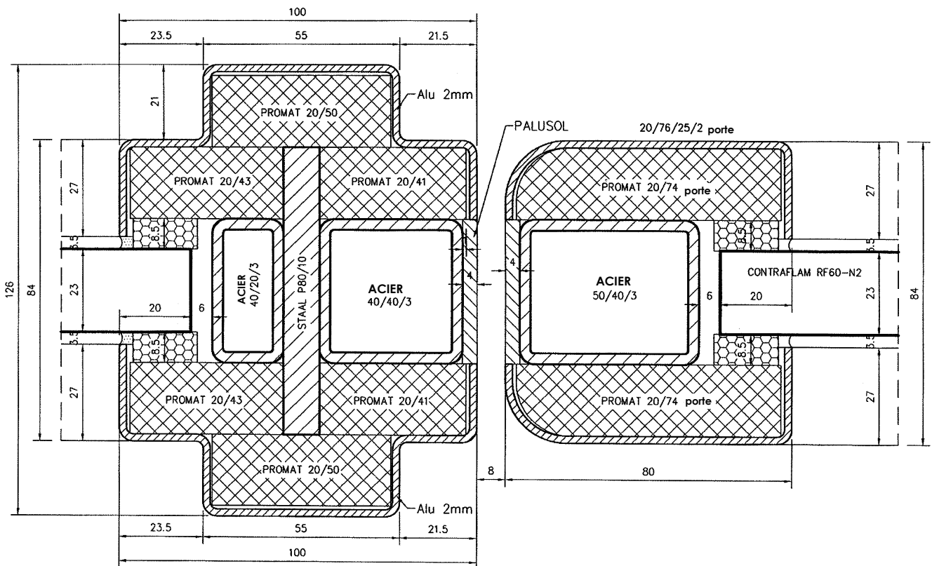
Détail C : Profilé de renfort vantail-panneau latéral/fenêtre
