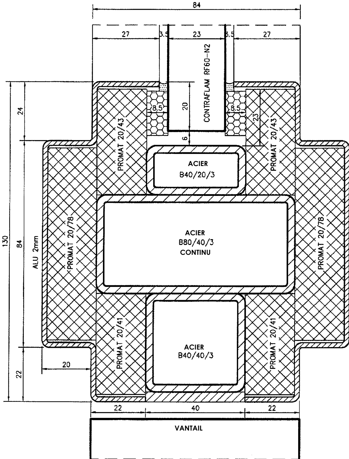
Détail A : Profilé de renfort vantail-imposte
