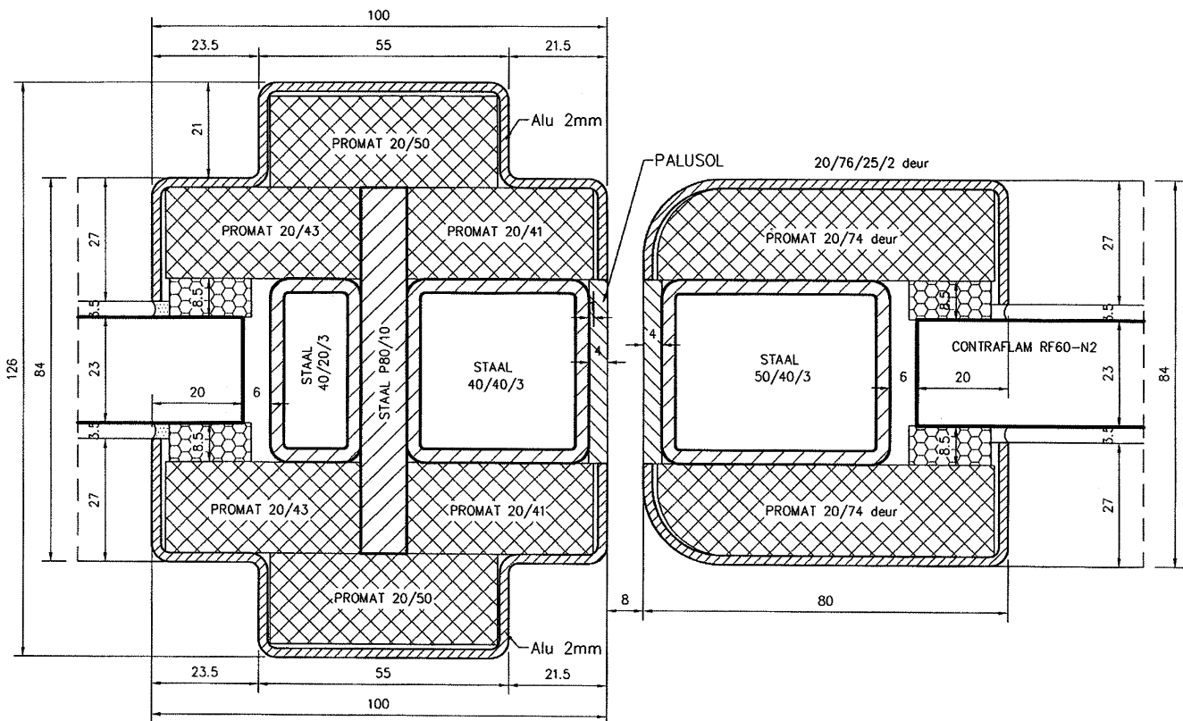
Detail C: Verstevigingsprofiel deurvleugel – zijpaneel/raam
