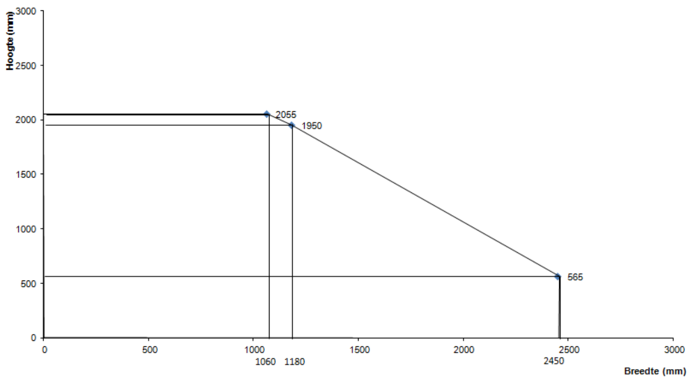
Figuur 5 Afmetingen AGC Pyrobel 25
