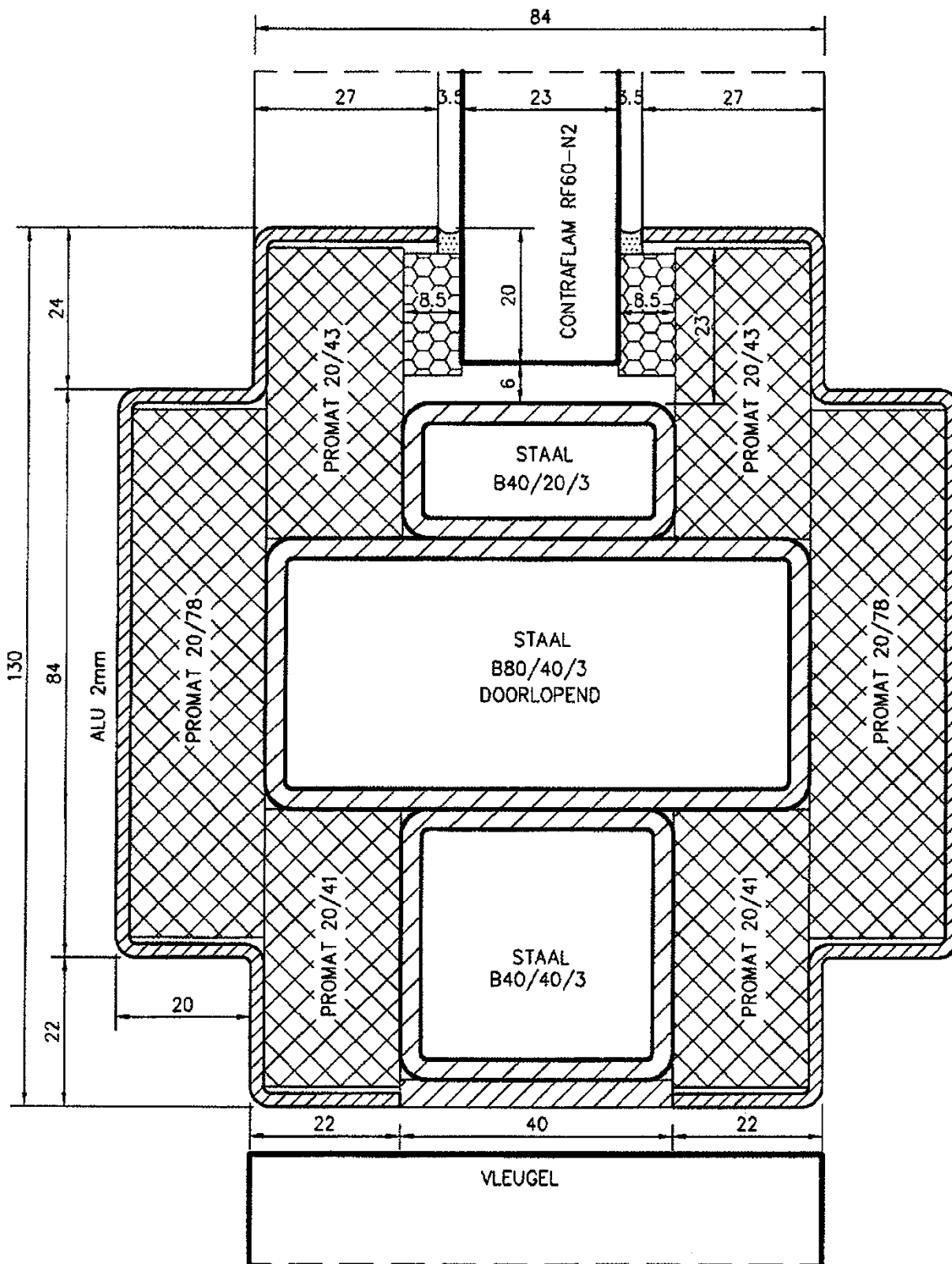
Detail A: Verstevigingsprofiel deurleugel – bovenpaneel
