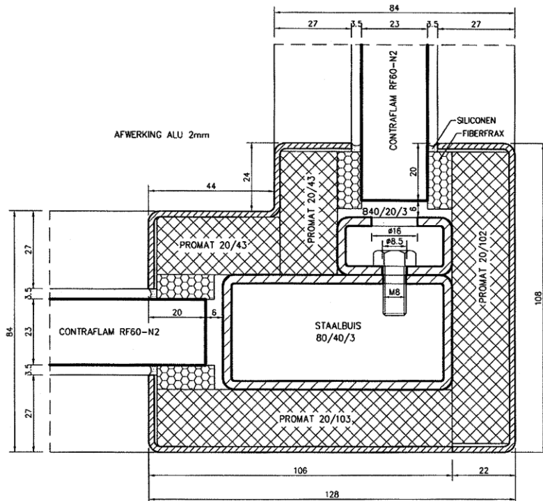
Detail D: Hoekverbinding raam (rechte hoek)
