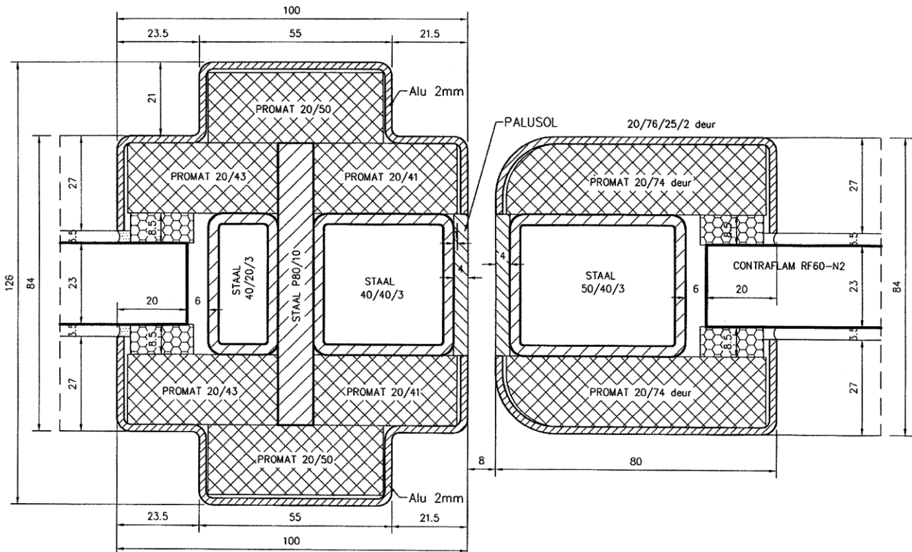
Detail C: Verstevigingsprofiel deurvleugel – zijpaneel/raam
