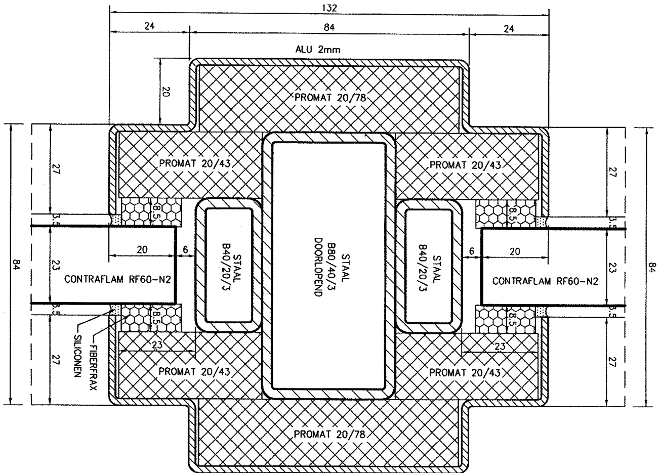
Detail B: Verstevigingsprofiel vaste beglazing
