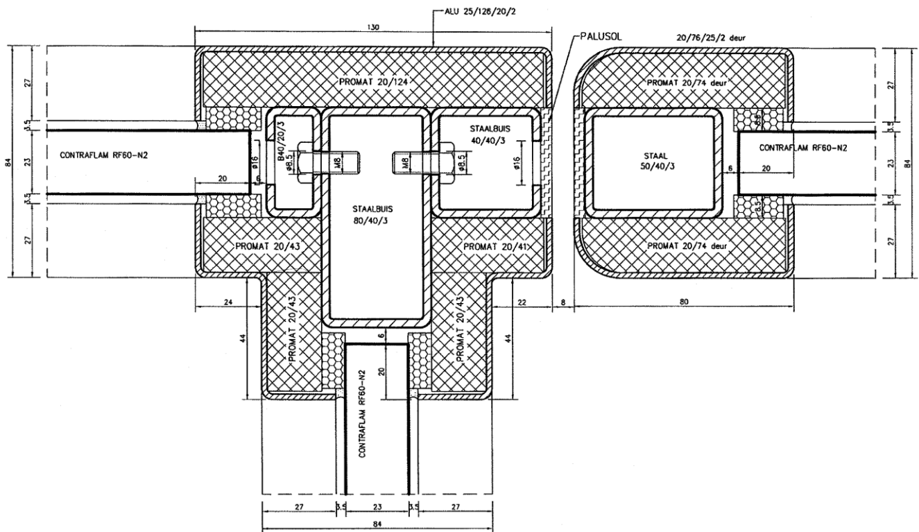
Detail F: Hoekverbinding t.p.v. deurvleugel (rechte hoek)
