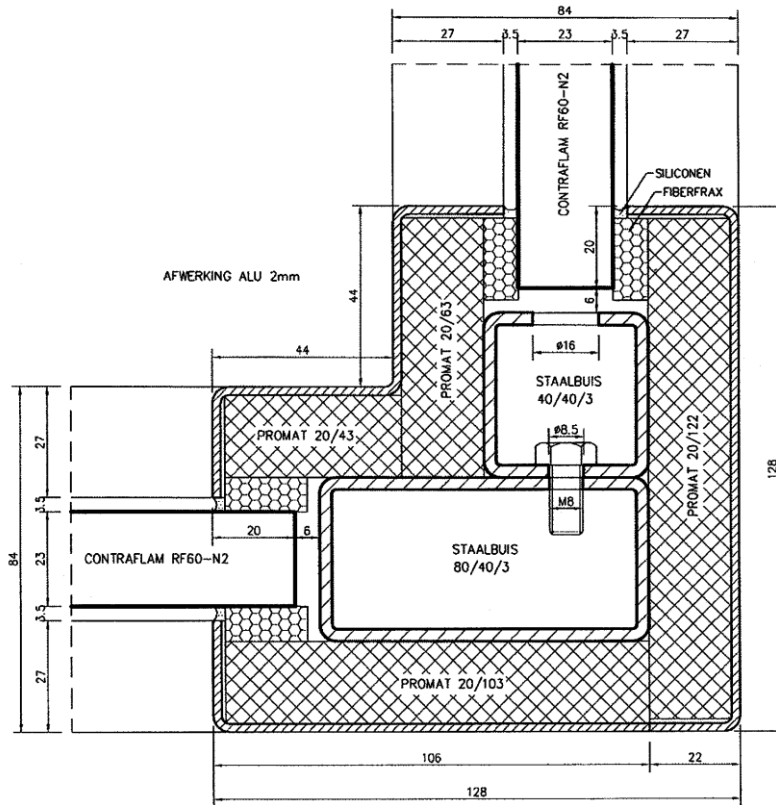
Detail D: Hoekverbinding raam (rechte hoek)
