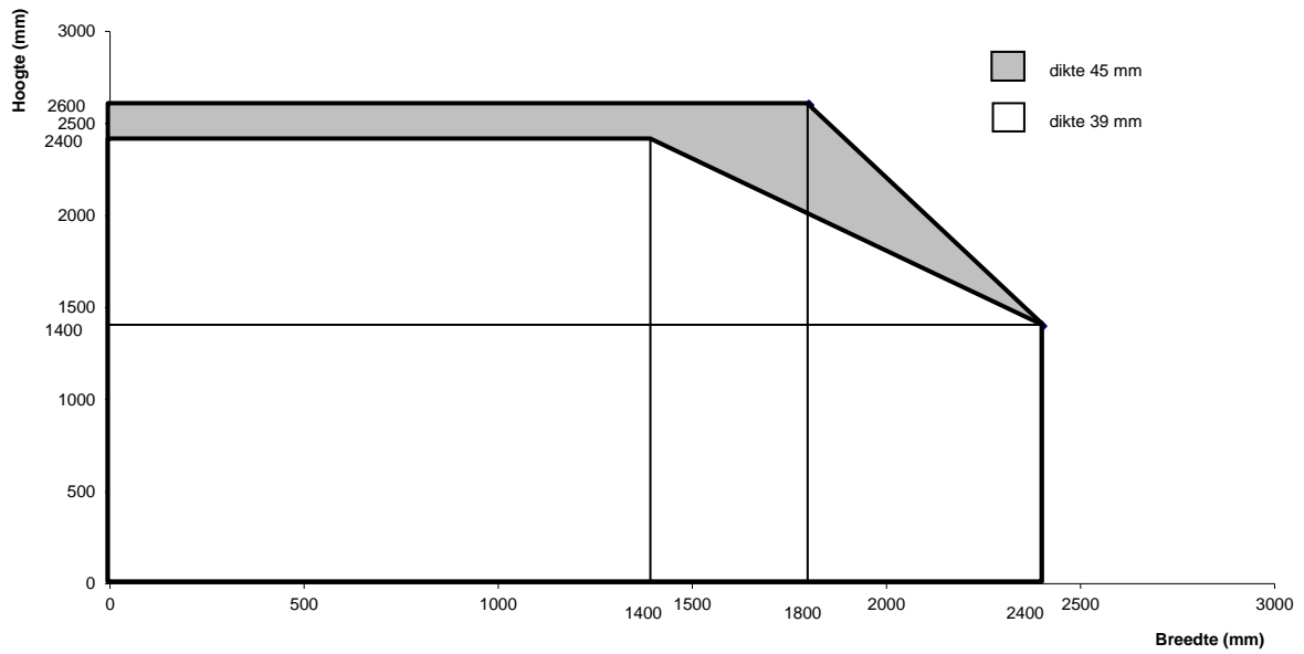
Afmetingen Contraflam 60 N2 ISO en Contraflam 60-3 ISO
