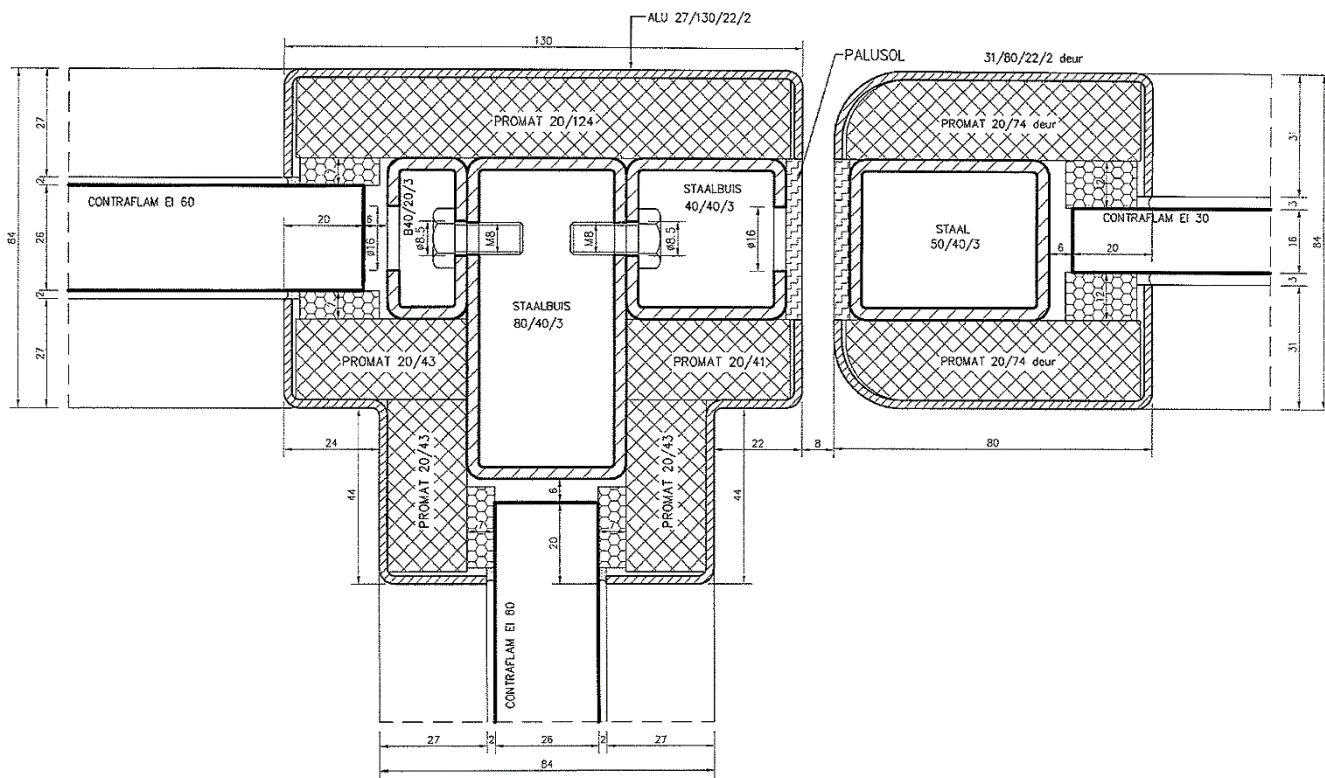
Detail 17: Hoekverbinding t.p.v. deurvleugel (rechte hoek)
