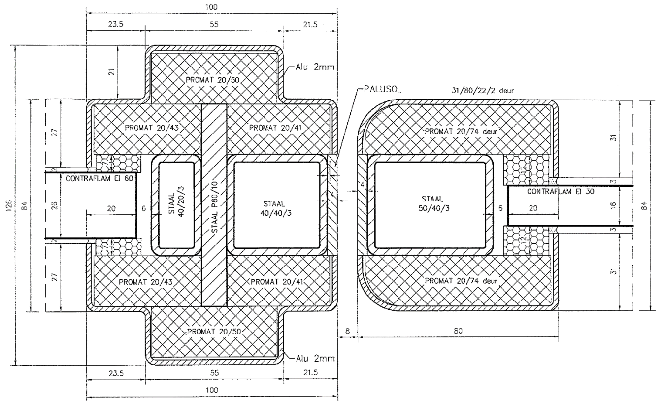
Detail 13: Verstevigingsprofiel deurvleugel – zijpaneel/raam
