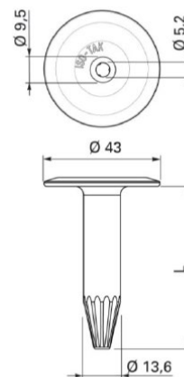
Fig. 5 – Bevestigingstule ISOTAK RP45
