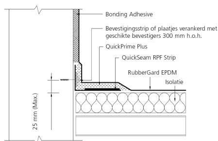
Fig. 16 – Kimfixatie met QS RPF Strip
