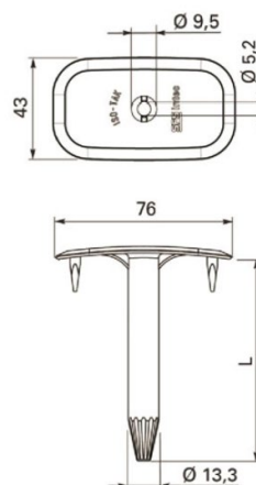
Fig. 4 – Bevestigingstule ISOTAK TWIN PEAK PLUS TPP 8040
