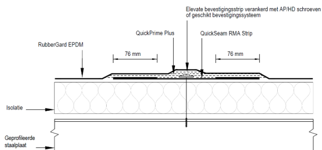
Fig. 14 – RMA Bevestigingssysteem
