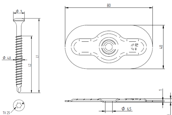
Fig. 10 – Schroef EUROFAST EDS-B 4,8 + bevestigingsplaatje EUROFAST DVP-EF-8040
