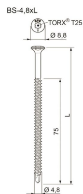
Fig. 3 – Schroef SFS Intec ISOTAK BS 48 +
