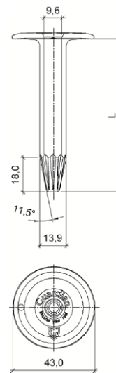
Fig. 9 – Bevestigingstule GUARDIAN R(P)45
