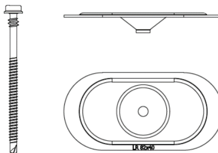
Fig. 11 – ETANCO EHB DF-2C 4.8+ bevestigingsplaatje ETANCO DVP DF 8240R
