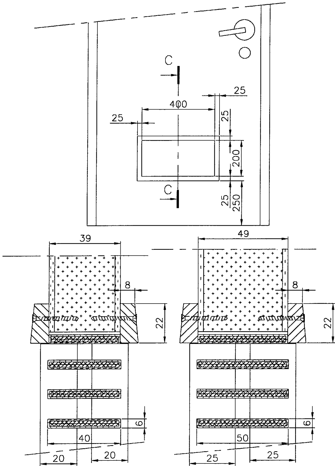
Snedes C-C
