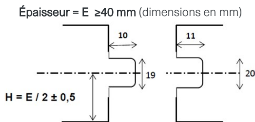
Figure 1 Dimensions rainure - languette pour Sopratherm Alu FW SJ et TMS
