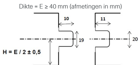
Fig. 1 – Afmetingen tand en groef van Sopratherm Alu FW SJ en TMS
