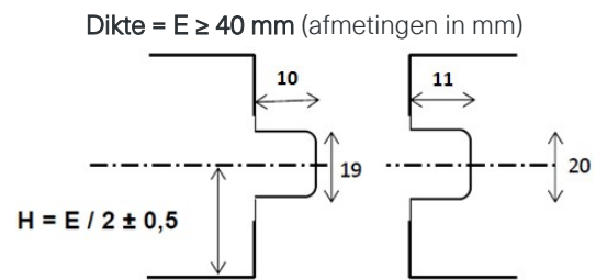
Figuur 1 Afmetingen tand en groef van Sopratherm Alu FW SJ en TMS
