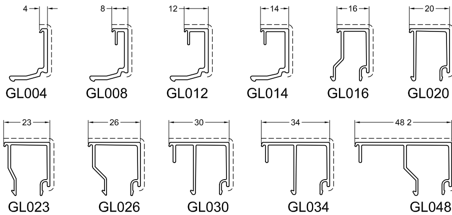
Figuur 9: glaslatten
