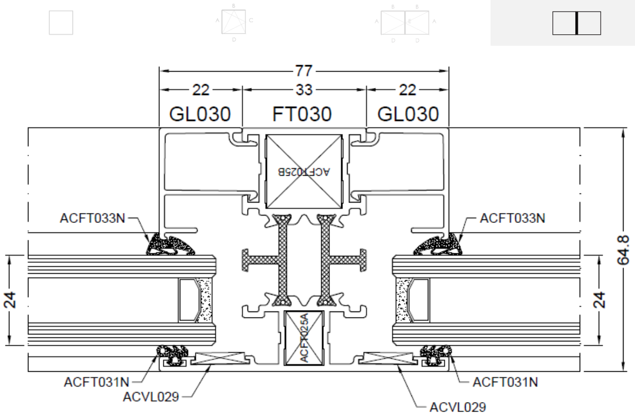
Figuur 4: Typesnede samengesteld venster
