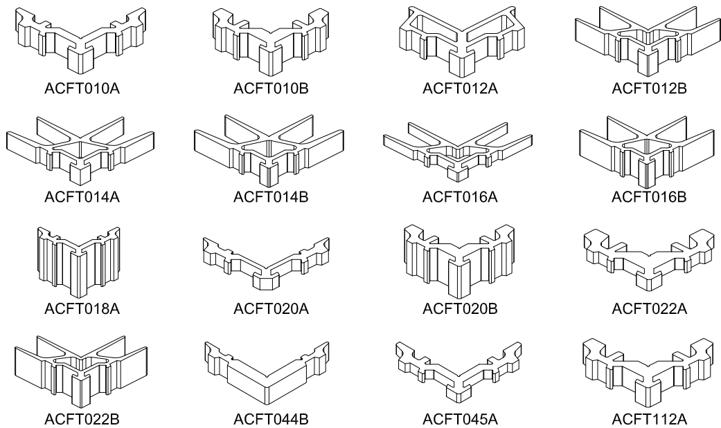
Figuur 11: pershoeken
