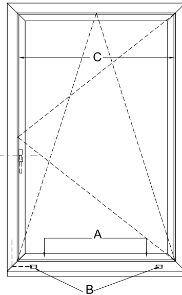
Figuur 17: draai-kipvenster, ontwatering en verluchting
