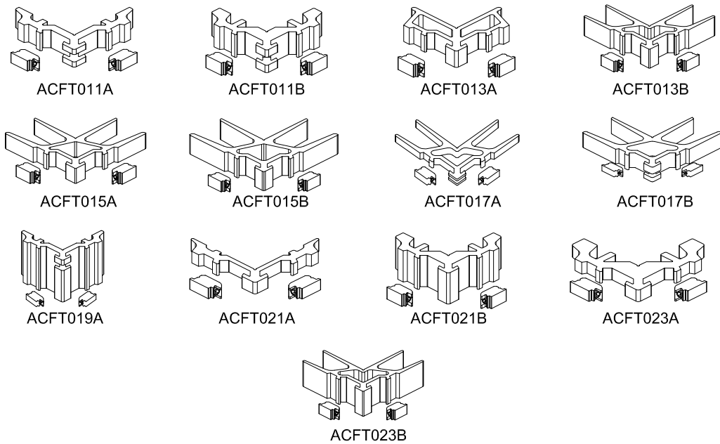
Figuur 11: pershoeken
