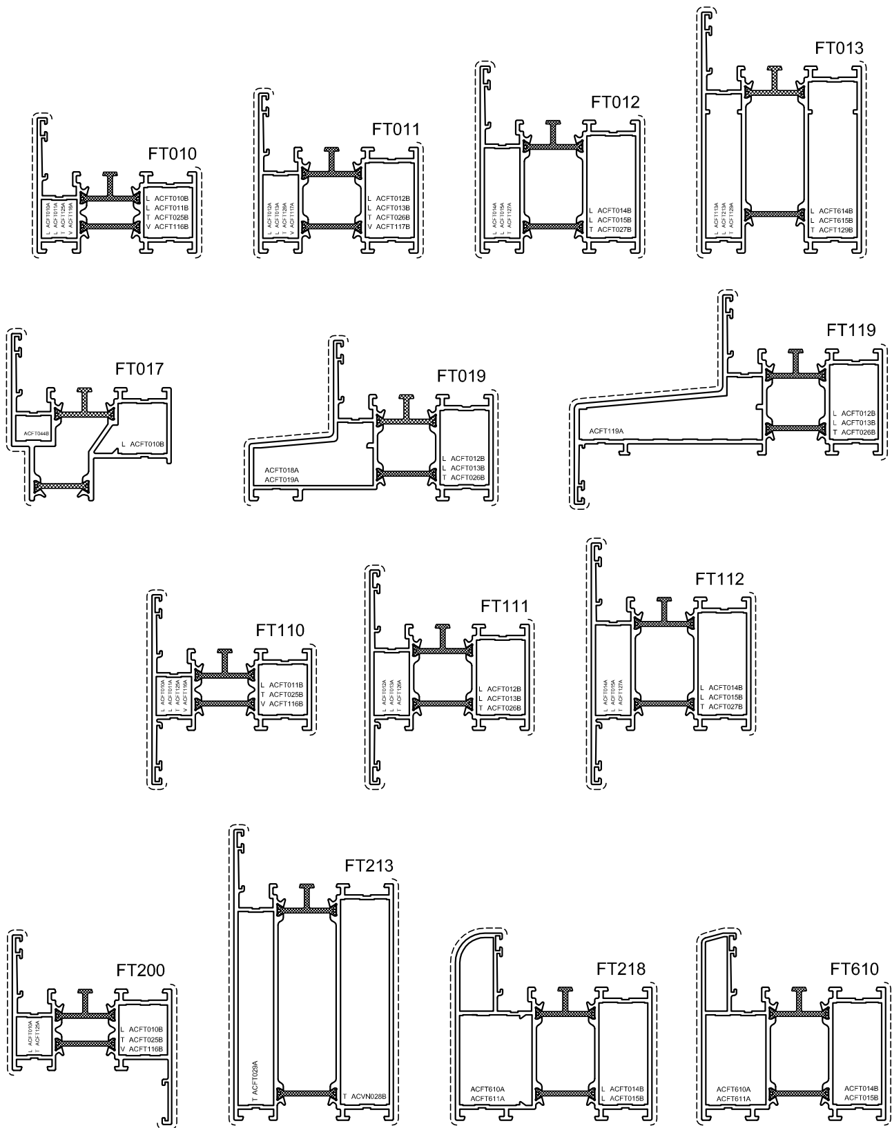
Figuur 1: vaste kaders
