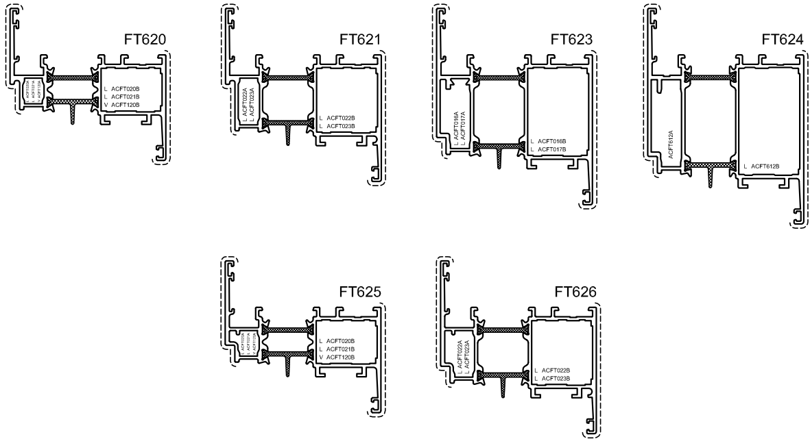
Figuur 3 (vervolg): vleugels
