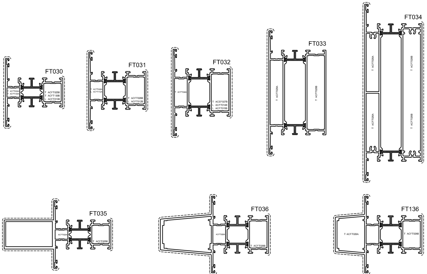
Figuur 4: stijlen en dwarsregels
