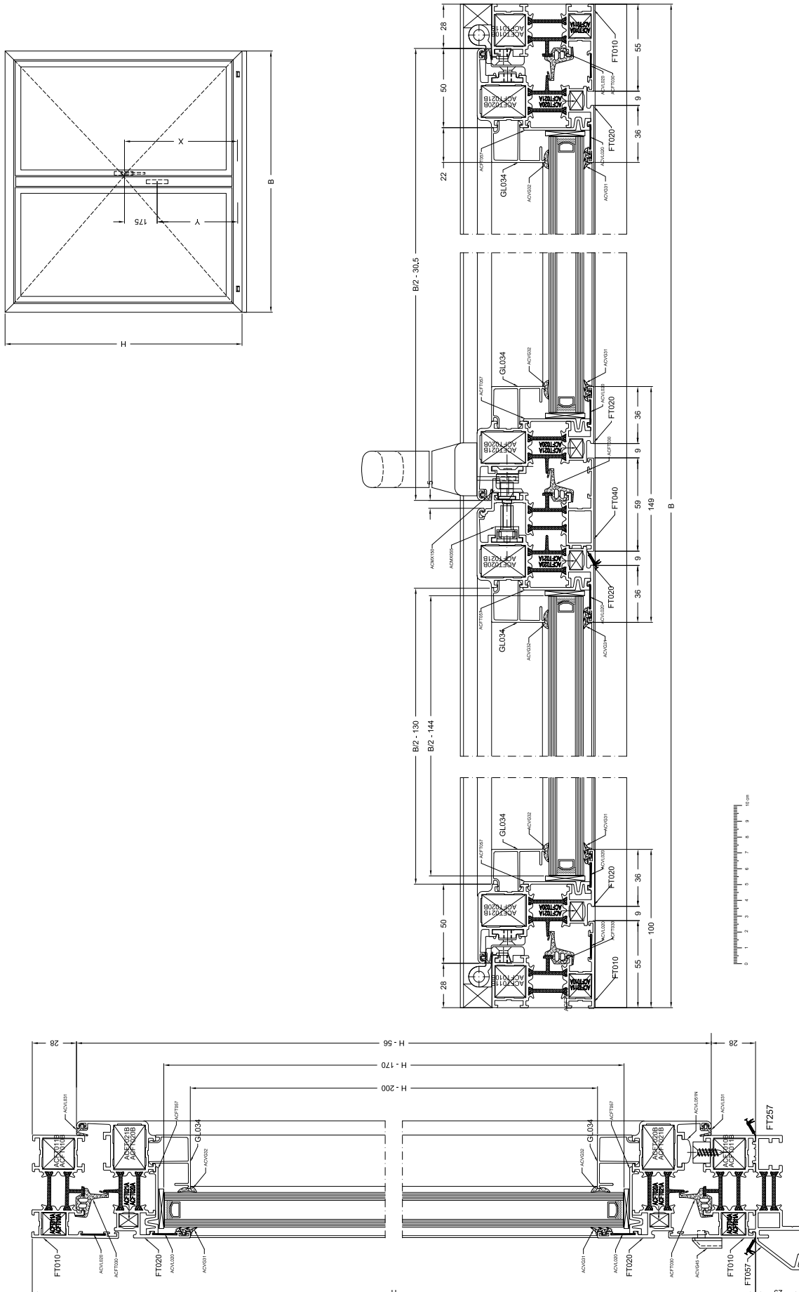
Figuur 16: stolpvenster
