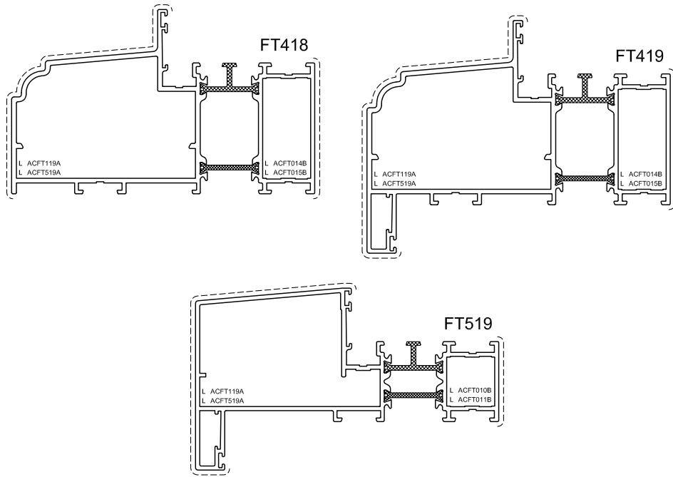
Figuur 3: vleugels
