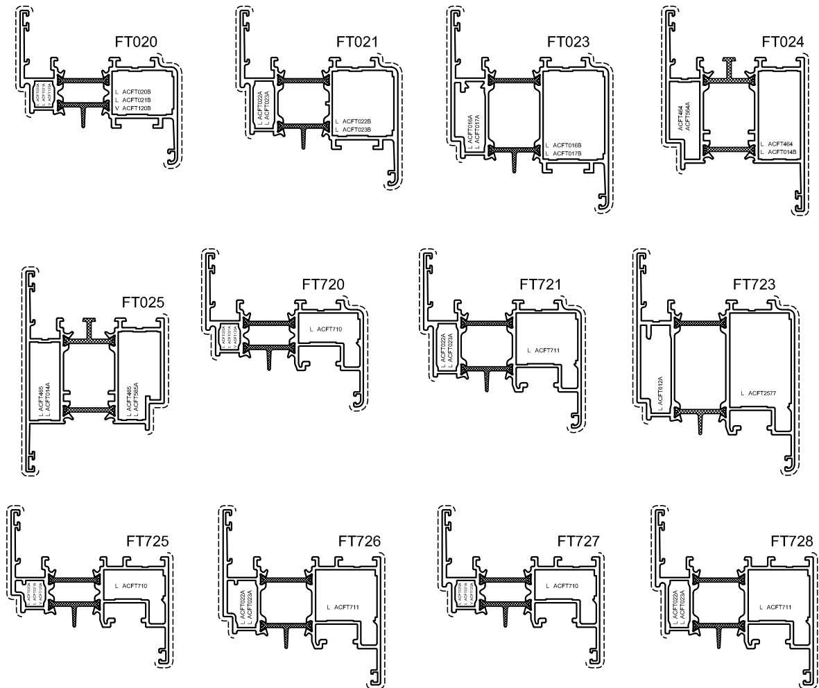
Figuur 3: vleugels
