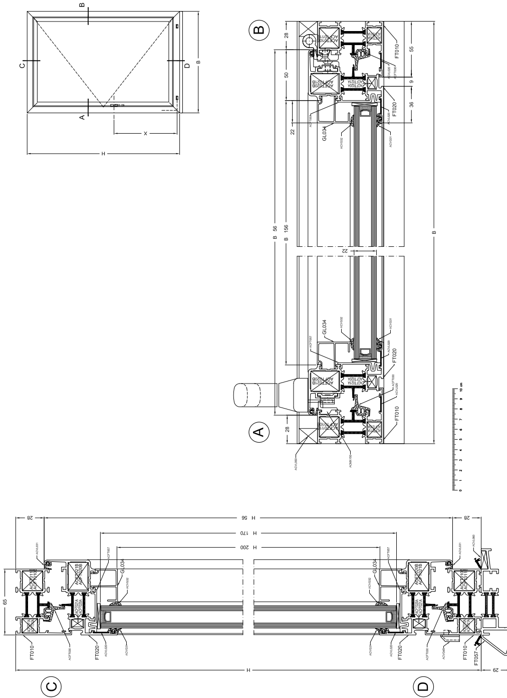
Figuur 15: draaivenster
