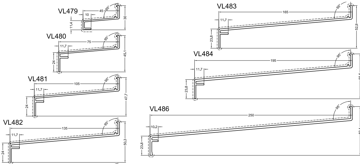
Figuur 9: glaslatten
