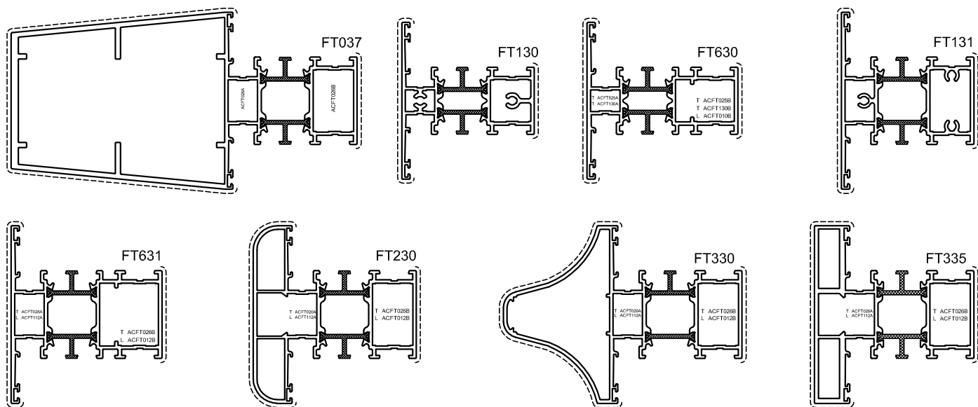
Figuur 4 (vervolg): stijlen en dwarsregels
