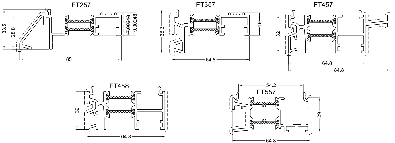
Figuur 8: dorpels
