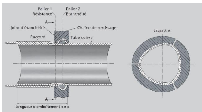
Fig. 3 coupe transversale pendant le sertissage avec une collerette à sertir
