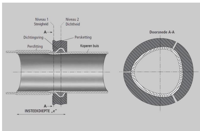
Fig. 3 dwarse doorsnede tijdens het inpersen (persketting)
