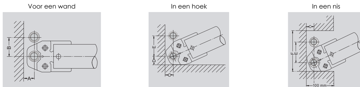
Fig. 4 benodigde vrije ruimte voor het inpersen
