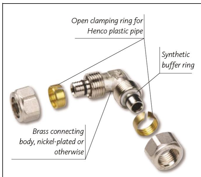
Fig. 2 Koppeling
