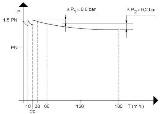
Fig. 3 Dichtheidscontrole
