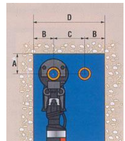
Espace libre requis pour le sertissage des manchons avec diamètres de 42 à 108 mm
