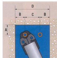
Vrije ruimte nodig voor het persen van moffen met een diameter van 12 tot 35 mm.
