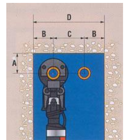
Vrije ruimte nodig voor het persen van moffen met een diameter van 42 tot 108 mm.
