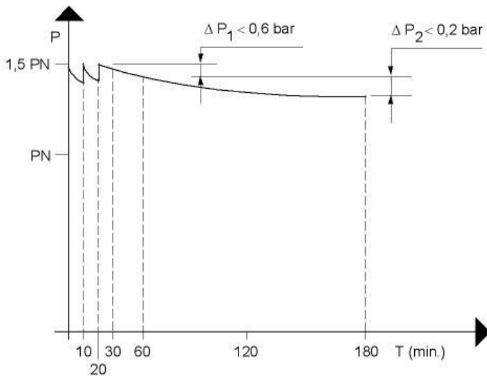
Fig. 2: Procedure dichtheidscontrole
