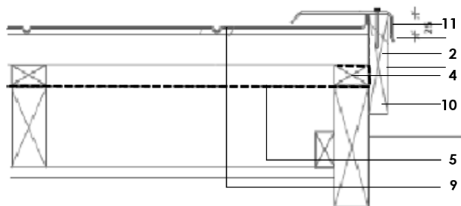
Fig. 12 – QUBE (ACOUSTIC) dakpannen – uitvoering van de dakvoet met dakvoetprofiel
