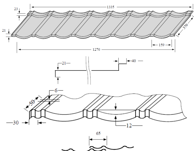
Fig. 1– METROTILE® BOND-dakpan
