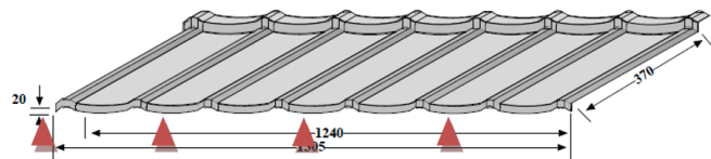
Fig. 24– METROTILE® ELEGANTA dakpan - plaatsing van de bevestigingen
