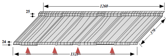
Fig. 21– METROTILE® SHAKE dakpan - plaatsing van de bevestigingen
