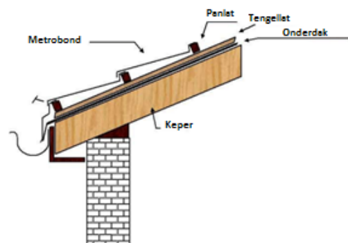
Fig. 25– METROTILE® BOND, METROTILE® BOND 7-PA, METROTILE® ROMAN, METROTILE® CLASSIC, METROTILE® SHAKE, METROTILE® WOODSHAKE, METROTILE® MISTRAL, METROTILE® ROMANA, METROTILE® GALLO, METROTILE® ELEGANTA dakpan - uitvoering van de dakvoet
