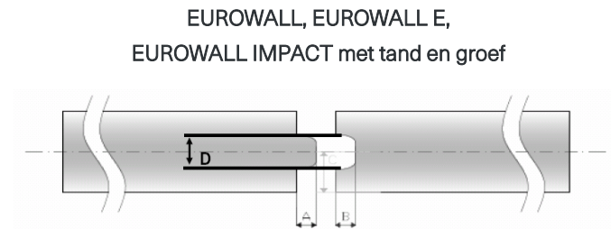
Fig. 1 – Tand en groef
