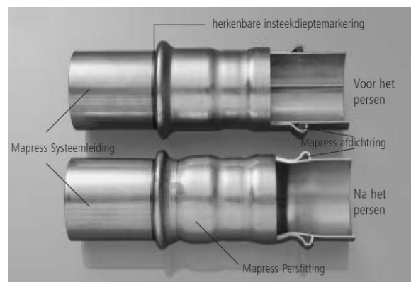
Fig. 1 – langse doorsnede vóór en na het inpersen
