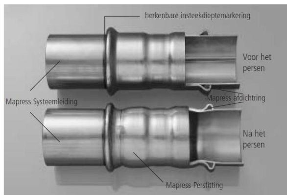
Fig. 1 langse doorsnede vóór en na het inpersen
