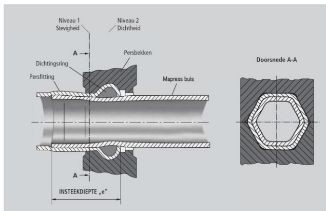
Fig. 2 dwarse doorsnede tijdens het inpersen (persklem)
