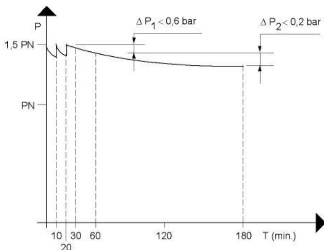
Fig. 5 procedure voor de dichtheidscontrole
