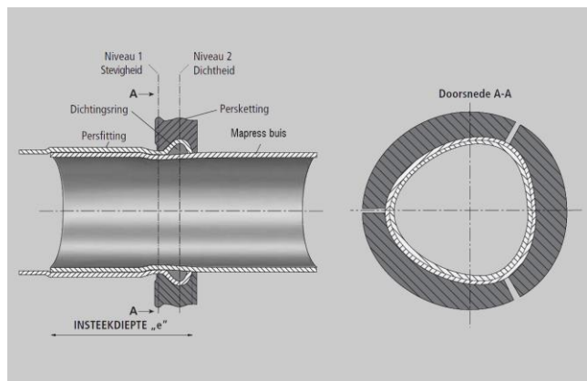
Fig. 3 dwarse doorsnede tijdens het inpersen (persketting)
