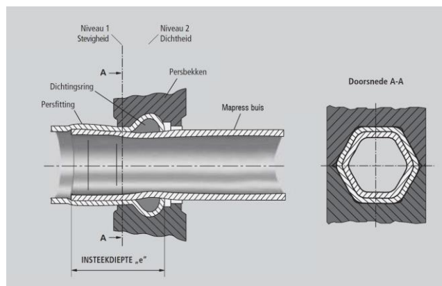
Fig. 2: dwarse doorsnede tijdens het persen (persklem)
