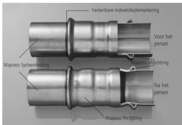
Fig. 1: langse doorsnede vóór en na het persen
