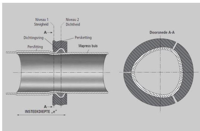
Fig. 3: dwarse doorsnede tijdens het persen (persketting)
