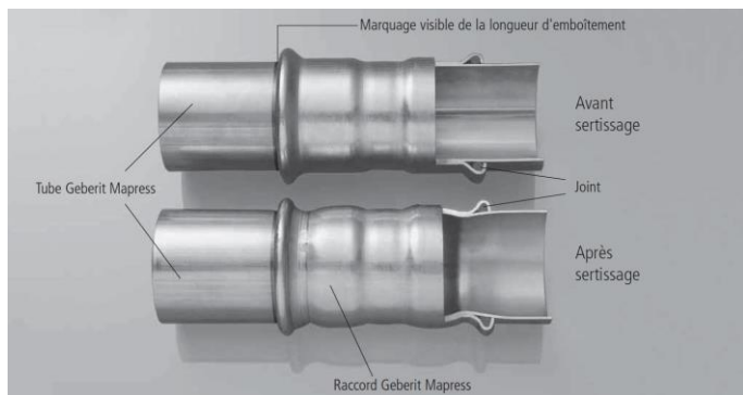
Fig. 1 coupe longitudinale avant et après le sertissage
