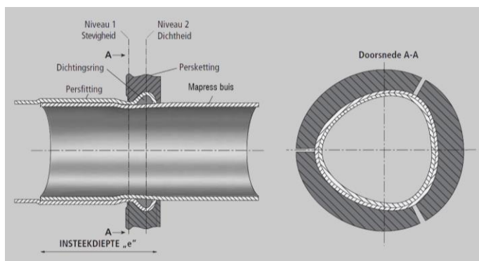
Fig. 3 dwarsdoorsnede tijdens het inpersen (persketting)
