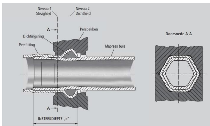
Fig. 2 dwarse doorsnede tijdens het inpersen (persklem)
