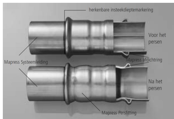
Fig. 1: langse doorsnede vóór en na het persen
