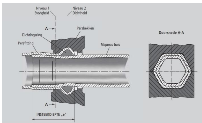
Fig. 2: dwarse doorsnede tijdens het inpersen (persklem)
