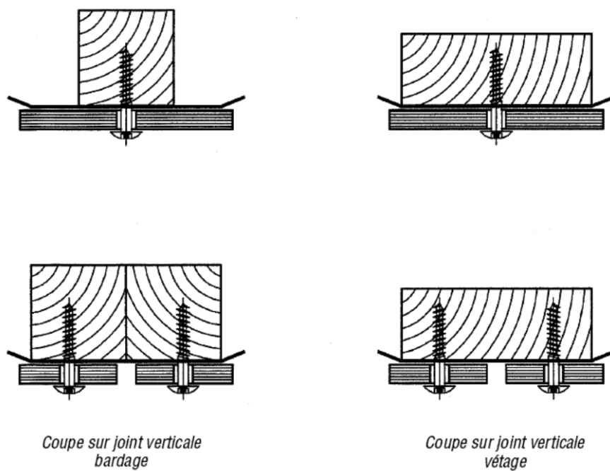
Figure 6 – Coupes
