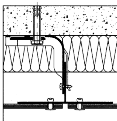
Fig. 3.4 – Joint vertical (vue en coupe horizontale)
