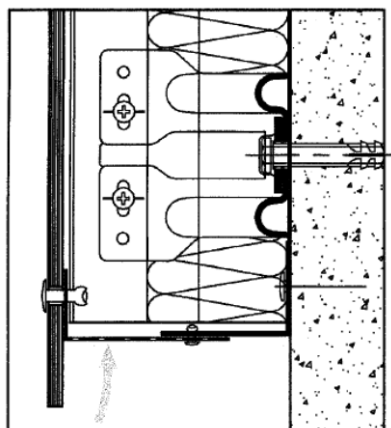
Fig. 3.3 – Finition de socle (vue en coupe verticale)
