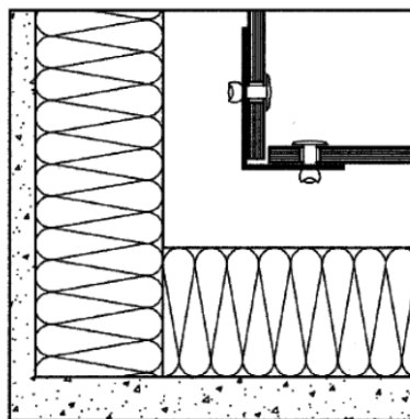
Fig. 3.6 – Angle intérieur (vue en coupe horizontale)
