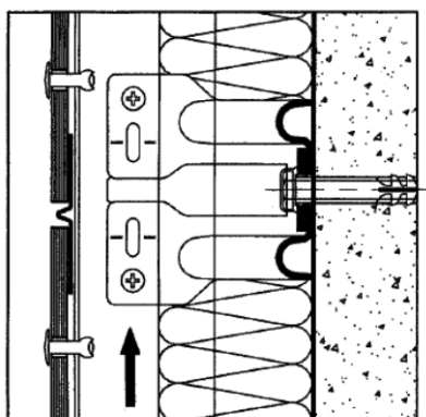
Fig. 3.3 – Finition de socle (vue en coupe verticale)
