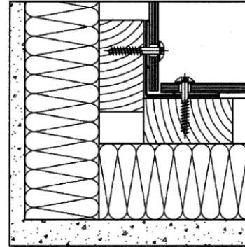
Fig. 2.6 – Binnenhoek (horizontale doorsnede)
