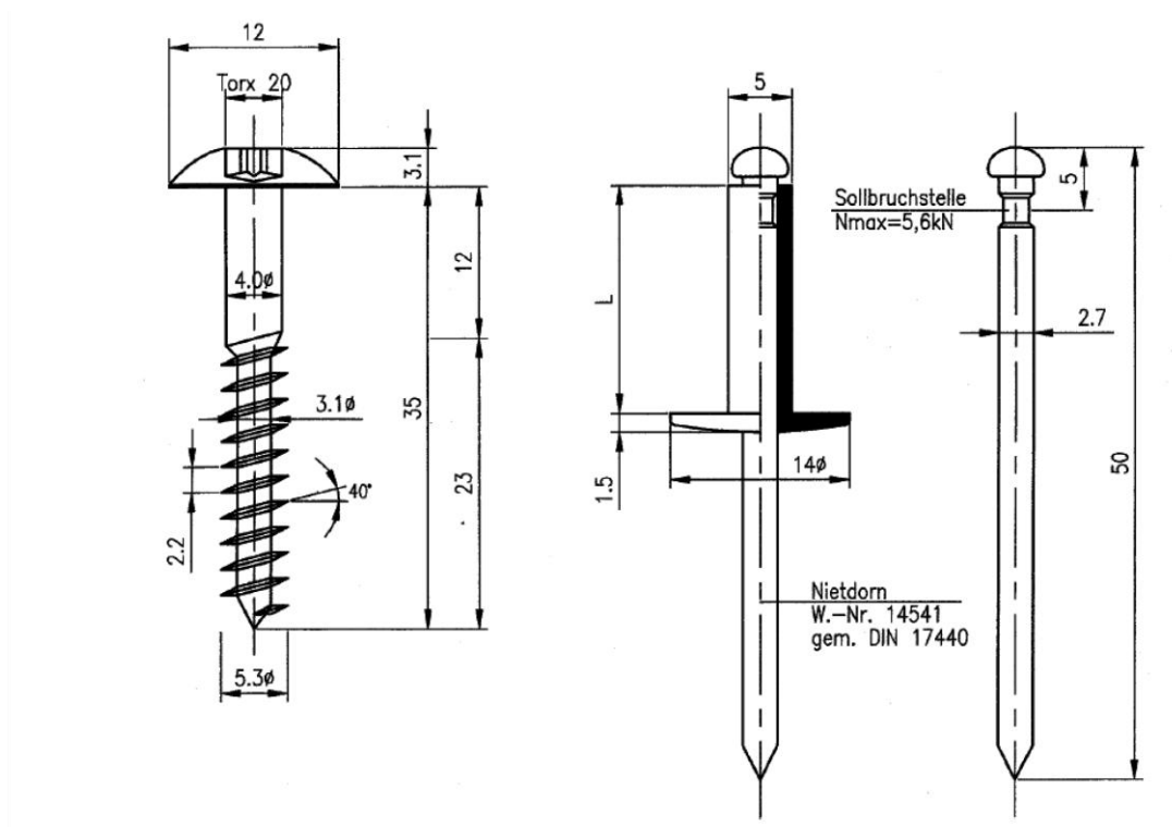
Figuur 1 - Bevestigingsmiddelen
