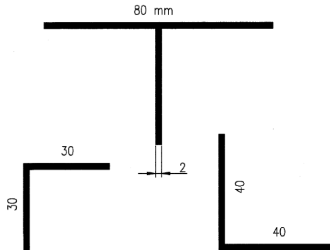
Figuur 3 - Doorsnedes in geval van stijl- en regelwerk uit aluminium
