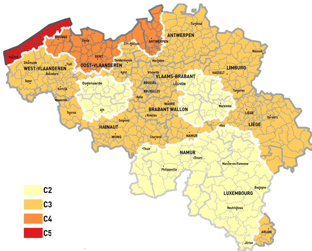
Figuur I.1- Corrosieklassen
