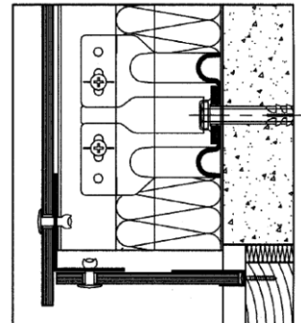
Fig. 3.4 – Verticale voeg (horizontale doorsnede)
