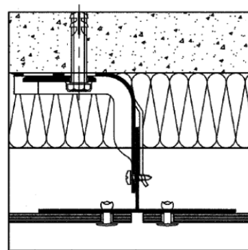
Fig. 3.6 – Binnenhoek (horizontale doorsnede)
