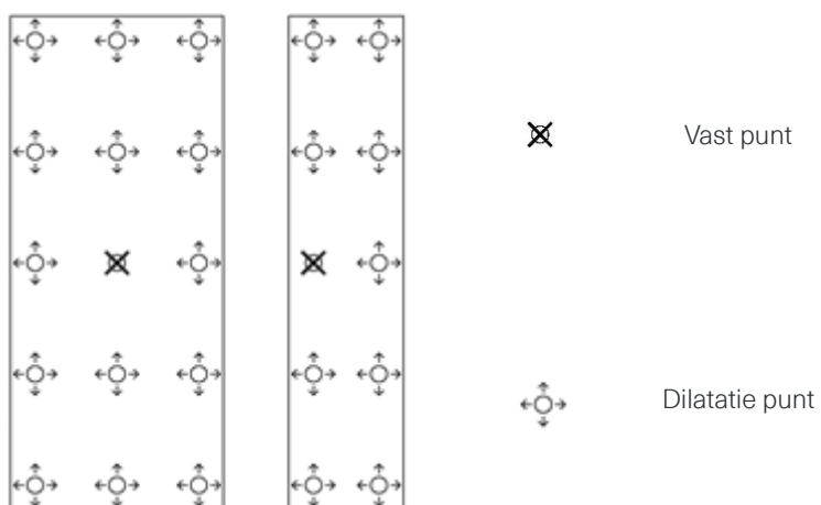
Figuur 7 – Principe van vast punt en dilatatiepunt
