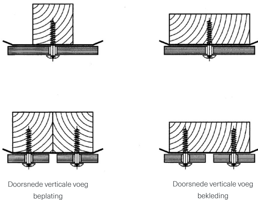
Figuur 6 - Doorsnedes
