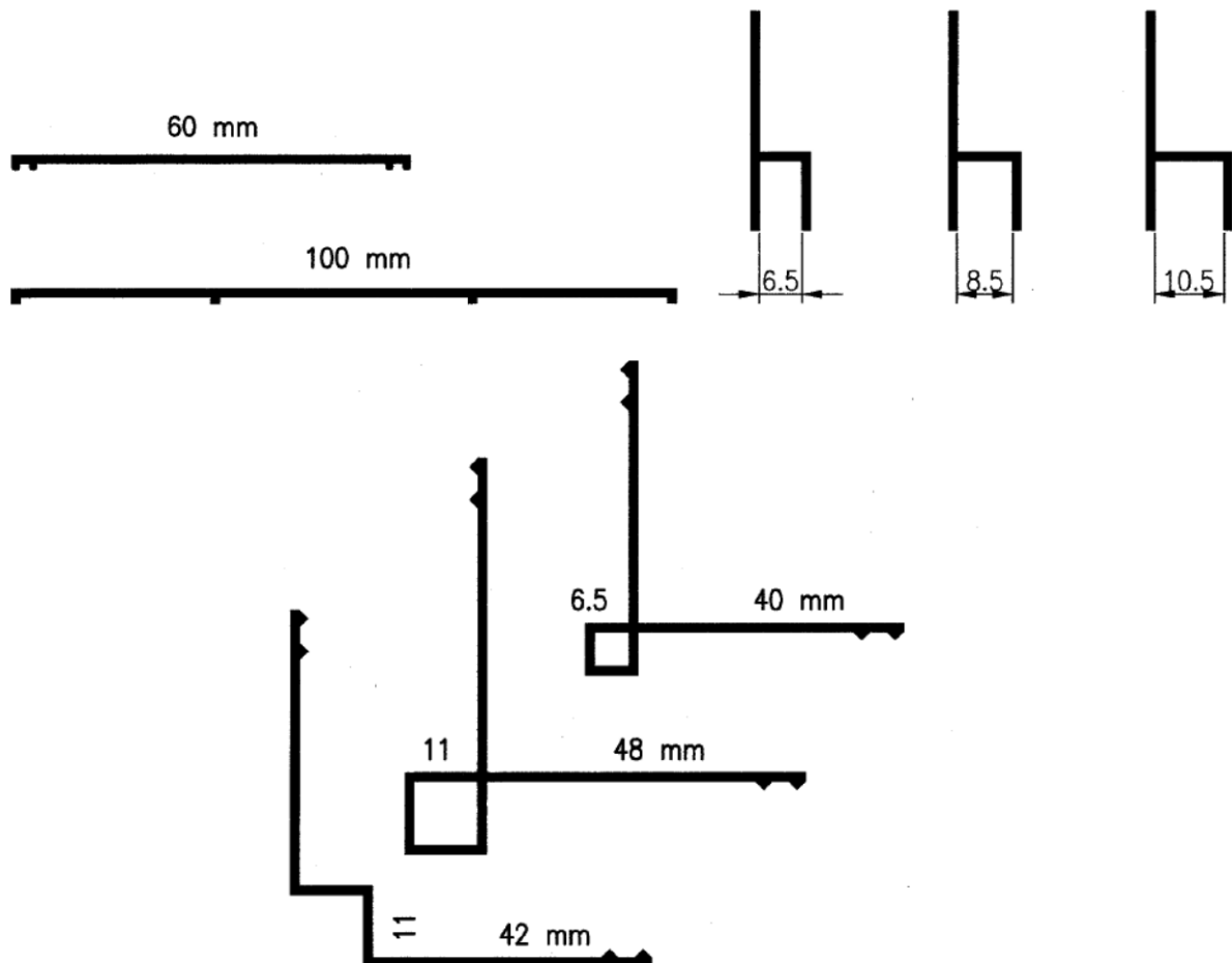
Figuur 5 - Voorbeelden van bijkomende profielen
