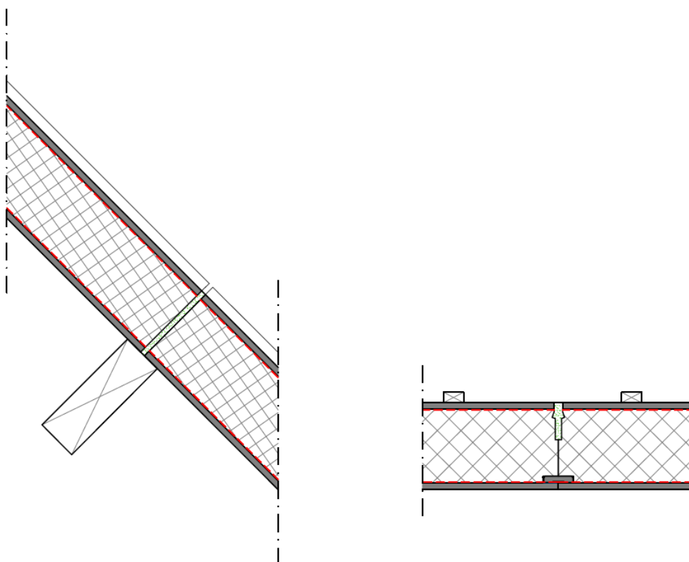
Fig. 2 Ussystem Roof SW Easy Airtight: voegen
