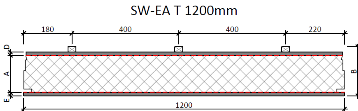
Fig. 1 Ussystem Roof SW Easy Airtight
