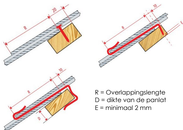
Fig. 2 – Bevestigingshaken: rechte haak, punthaak, klemhaak
