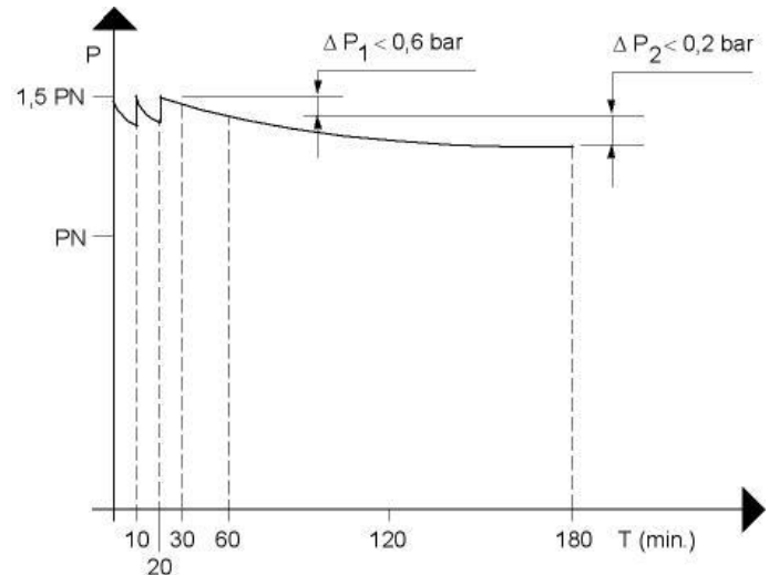
Fig. 2: Dichtheidscontrole
