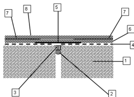
Fig. 1 – Opstand
