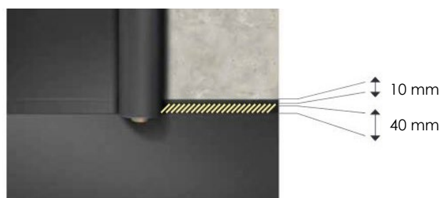
Fig. 4 – Langsnaden bij PRELASTI FLEECE voor losliggende en verkleefde systemen
