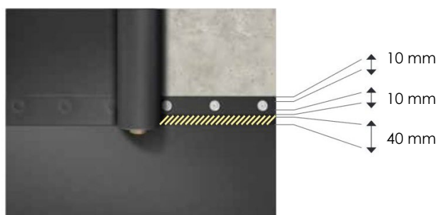
Fig. 5 – Langsnaden bij PRELASTI FLEECE voor mechanische bevestigde systemen
