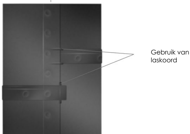
Fig. 6 – Langsnaden bij PRELASTI FLEECE voor mechanische bevestigde systemen
