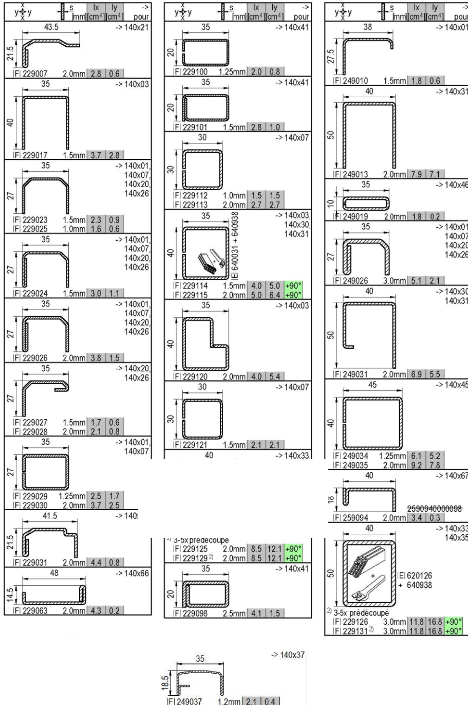
Figure 3: Profilés de renfort en acier galvanisé
