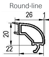
Figure 5 : Variantes d'exécution des parclozes
