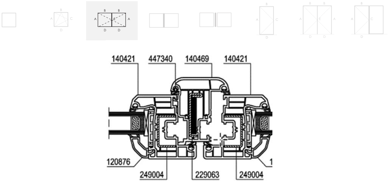
Figure 7c: Coupe-type de fenêtre à double ouvrant avec mauclair
