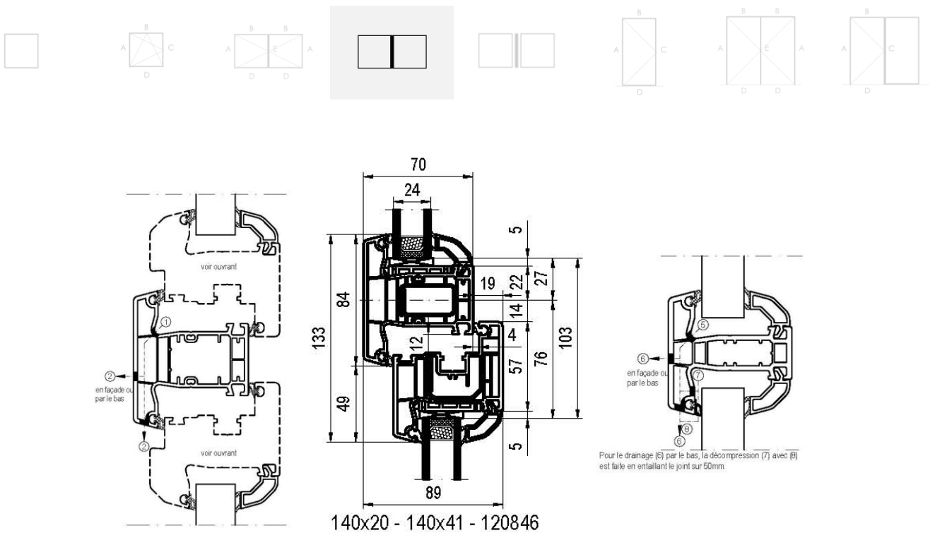
Figure 7d: Coupe-type de fenêtre composée
