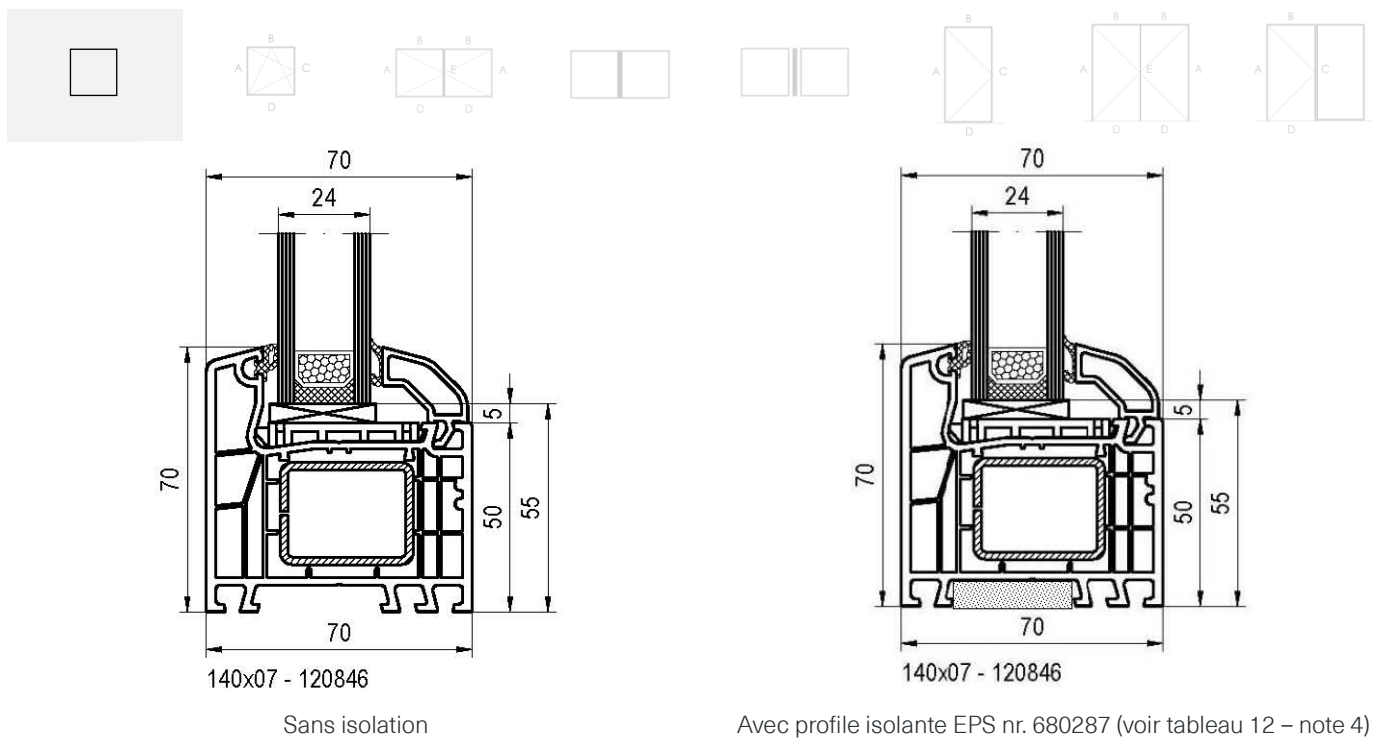
Figure 7a: Coupe-type de fenêtre fixe
