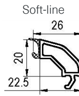
Figure 5 : Variantes d'exécution des parclozes
