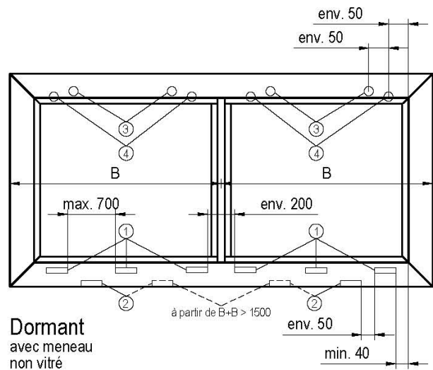
Figure 8: Drainage et décompression
