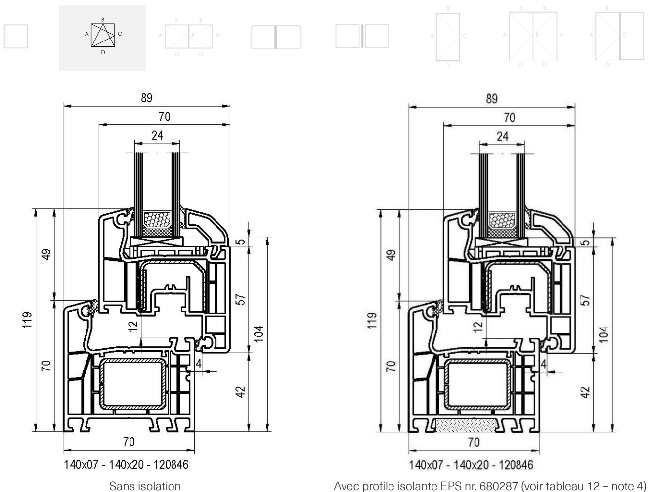
Figure 7b: Coupe-type de fenêtre oscillo-battante
