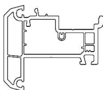
Figuur 3: Versterkingsprofielen uit gegalvaniseerd staal
