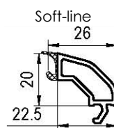
Figuur 5: Uitvoeringsvarianten glaslatten
