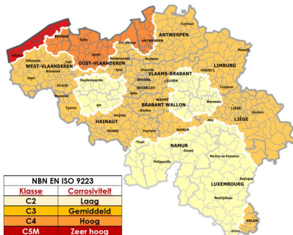
Figuur 1: Geografische agressiviteitszones (prSTS 71-2)
