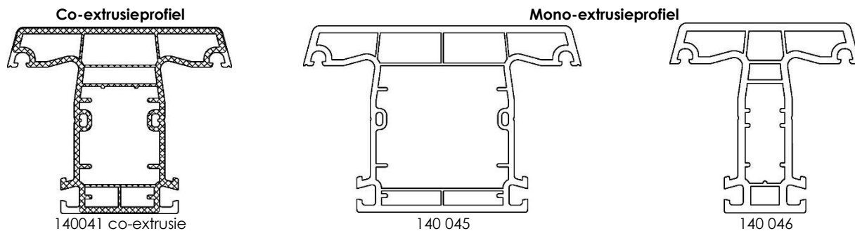
Figuur 2c: Tussenstijlen en dwarsregels
