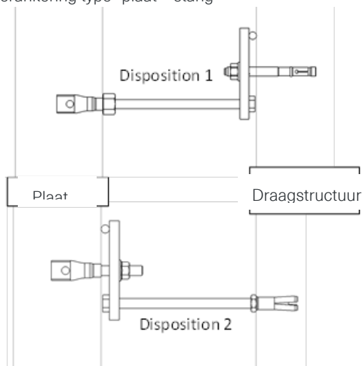
Windverankering type "plaat + stang"
