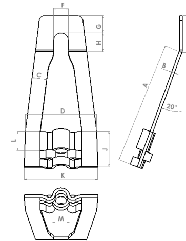
Gewone plaat voor de categorieën van 5,0 tot 35,0 kN
