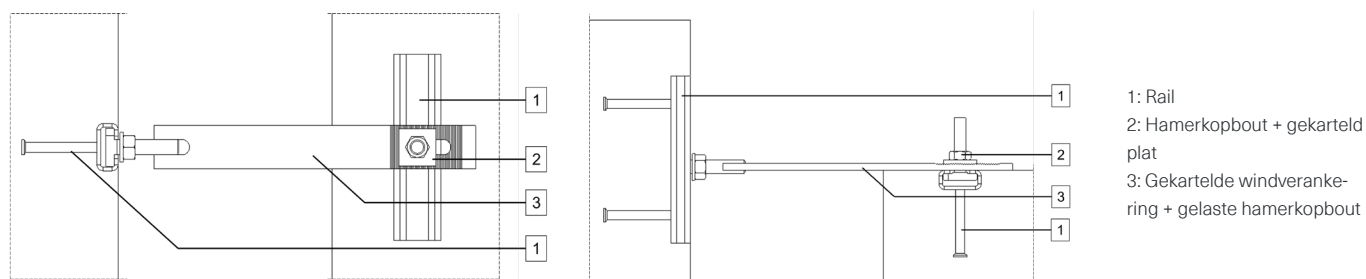
Windverankering van kanten met U- sectie d.m.v. platverbinding met hamerkopbout
