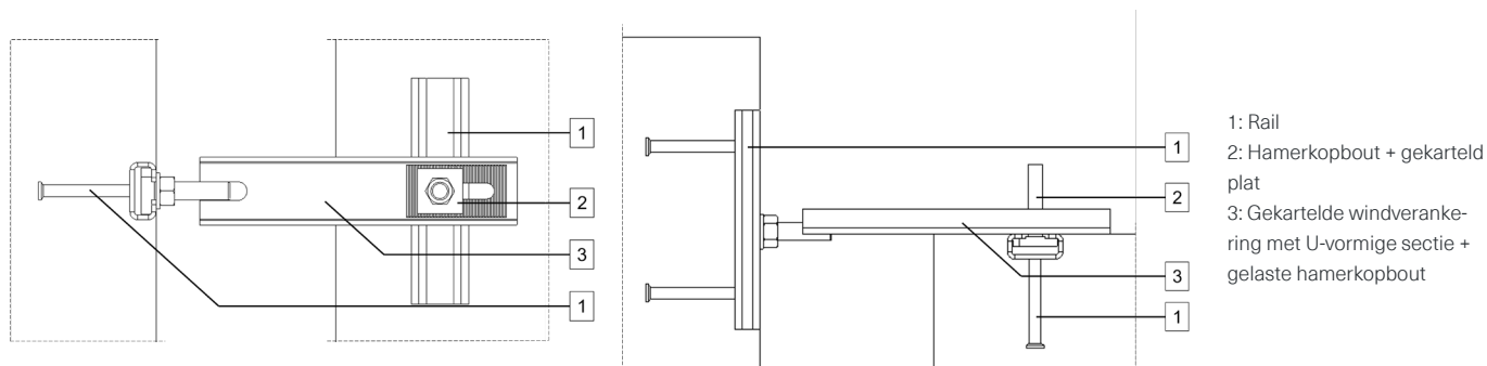
Windverankering van kanten met U- sectie d.m.v. platverbinding met hamerkopbout
