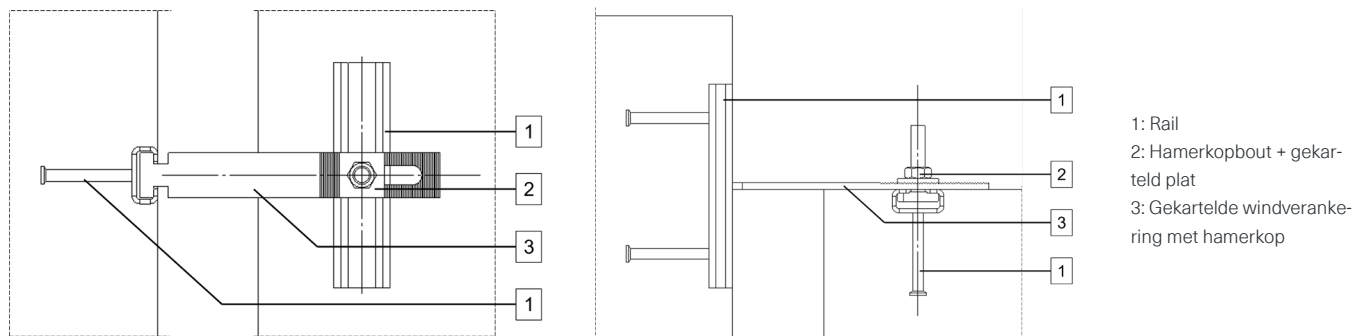
Windverankering van kanten d.m.v. platverbinding met hamerkopbout
