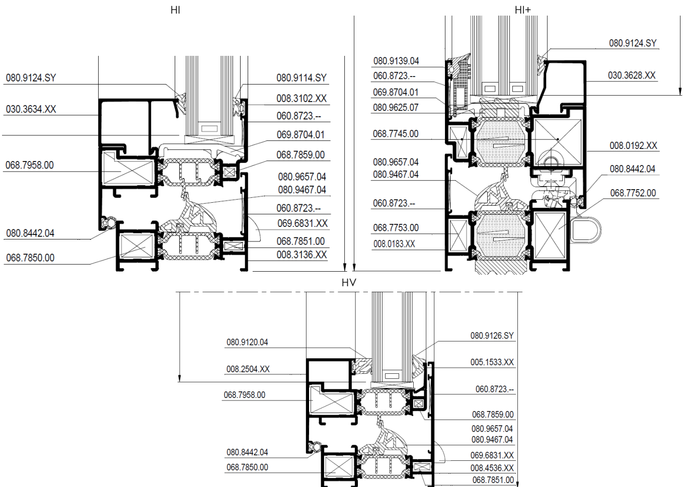
Figuur 2: Uitvoeringsvarianten venstervleugel
