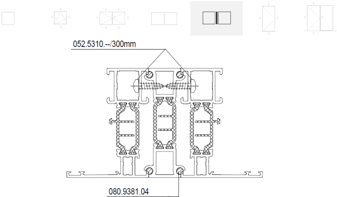
Figuur 8: Typesnede schrijnwerkgeheel
