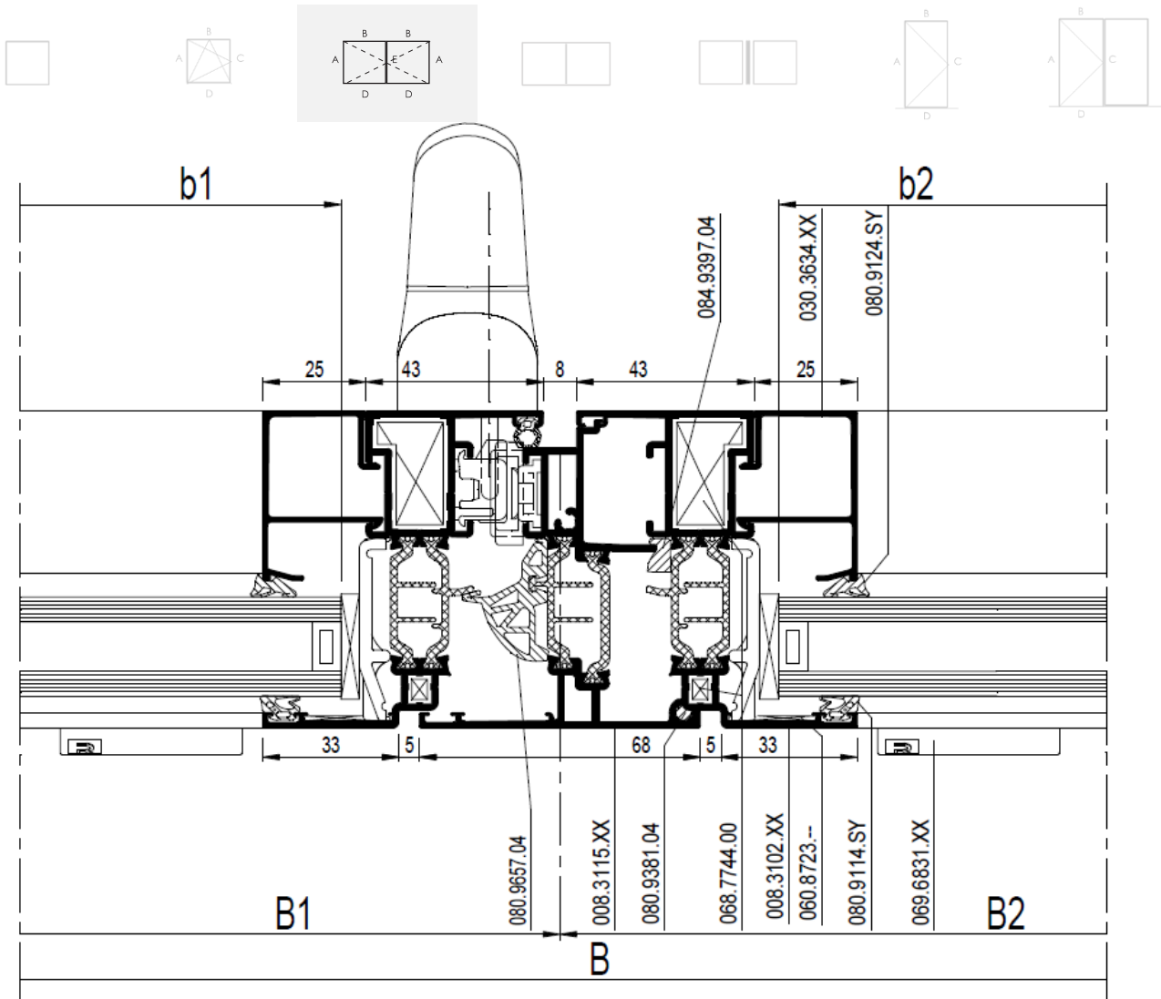
Figuur 6: Typesnede stolp venster
