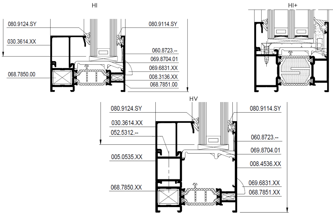
Figuur 1: Uitvoeringsvarianten vast kader
