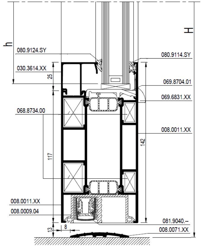
Dorpelprofil, met sokkelprofiel
