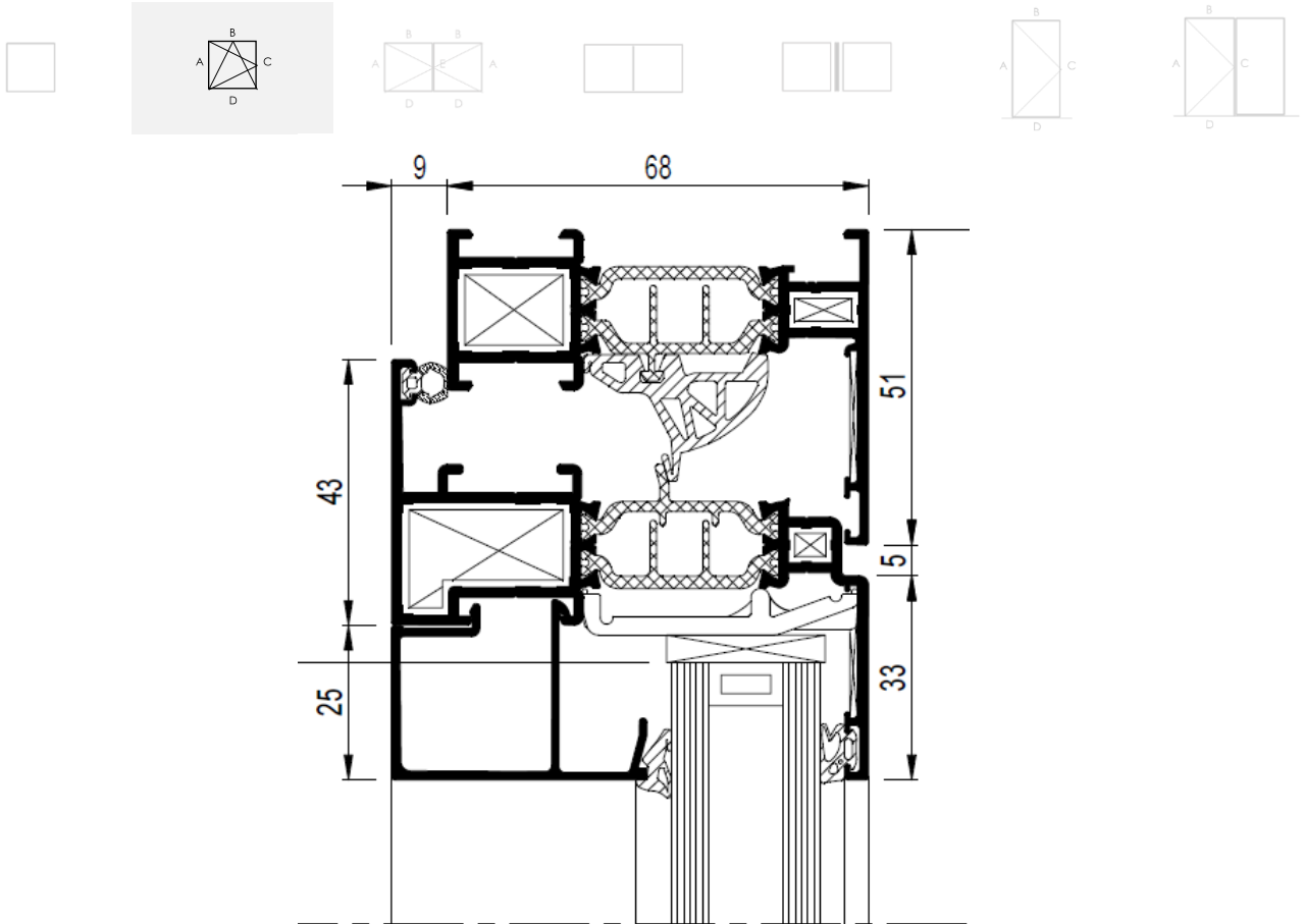
Figuur 5: Typesnede draai-kip venster
