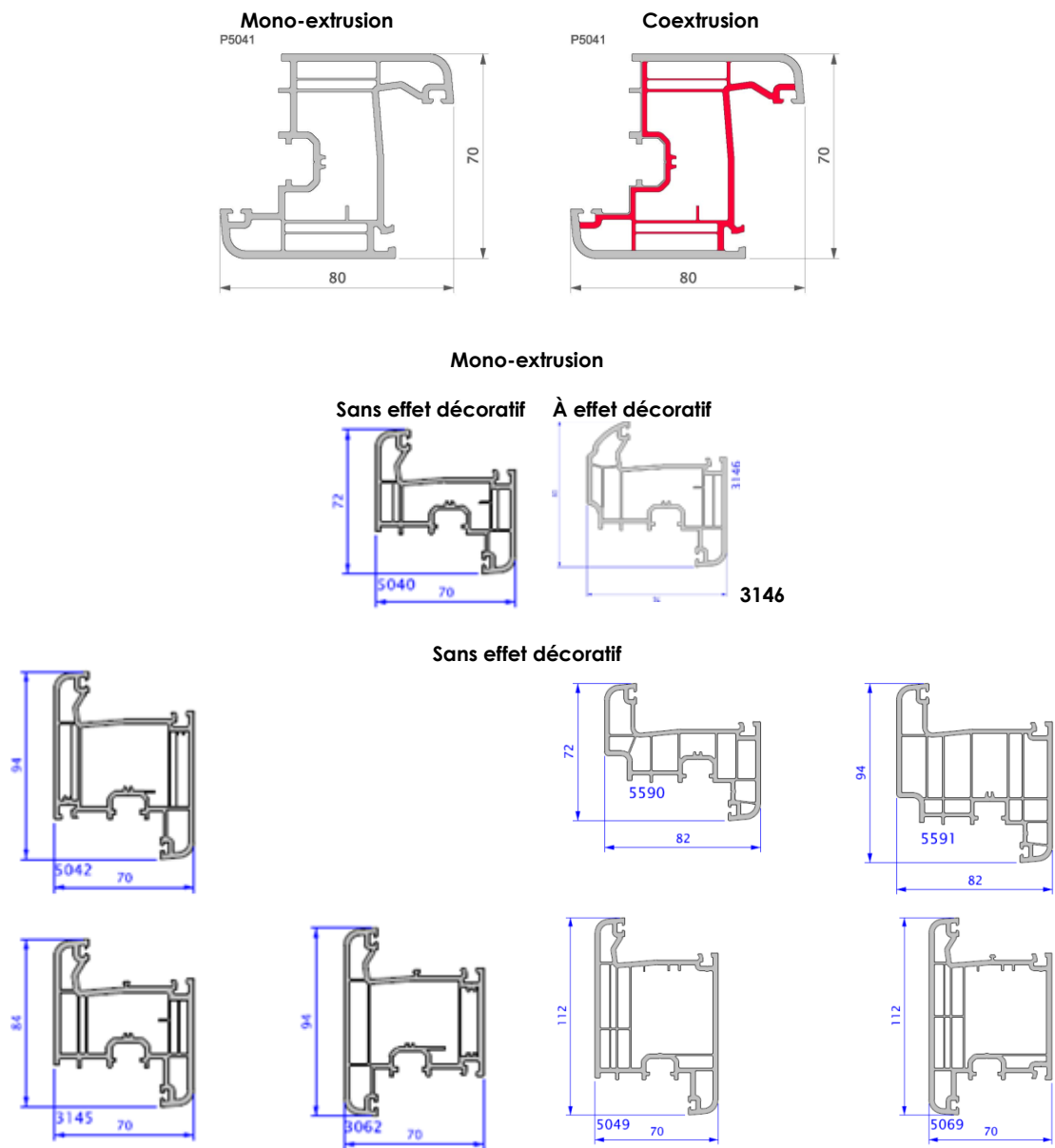
Figure 2b: Profilés d'ouvrant
