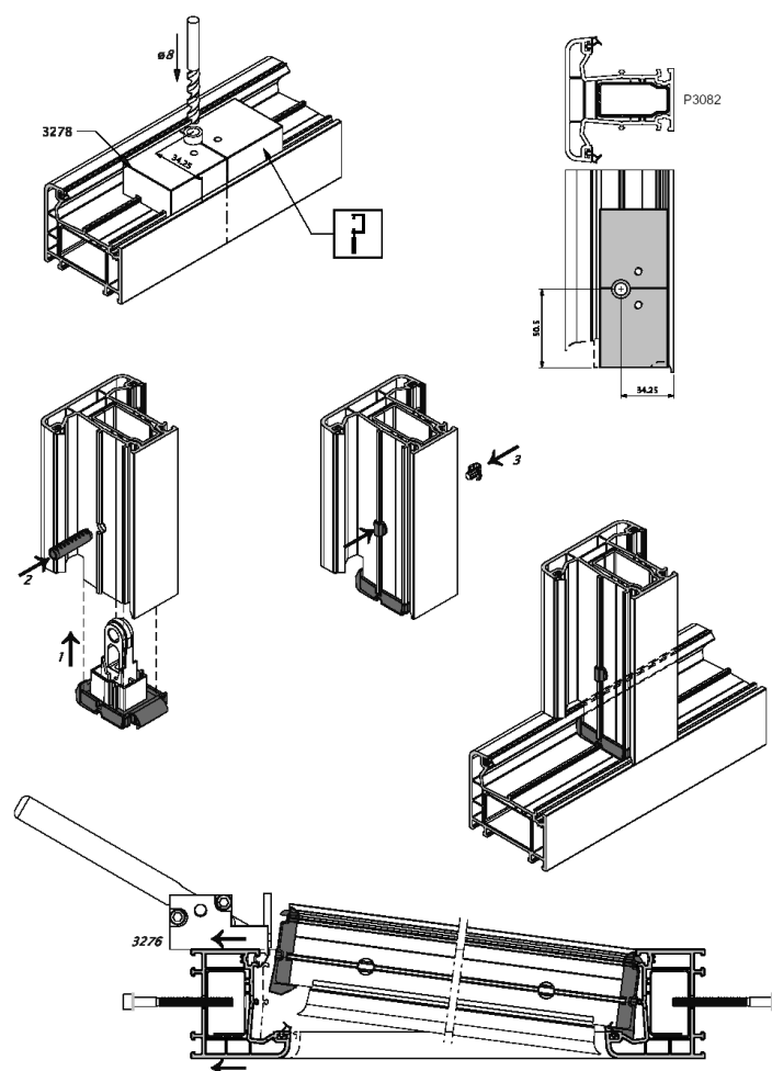
Figure 2d: Assemblage mécanique en T avec boulon d'entretoisement
