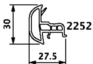
Figuur 5b: Makelaar als hulppofiel
