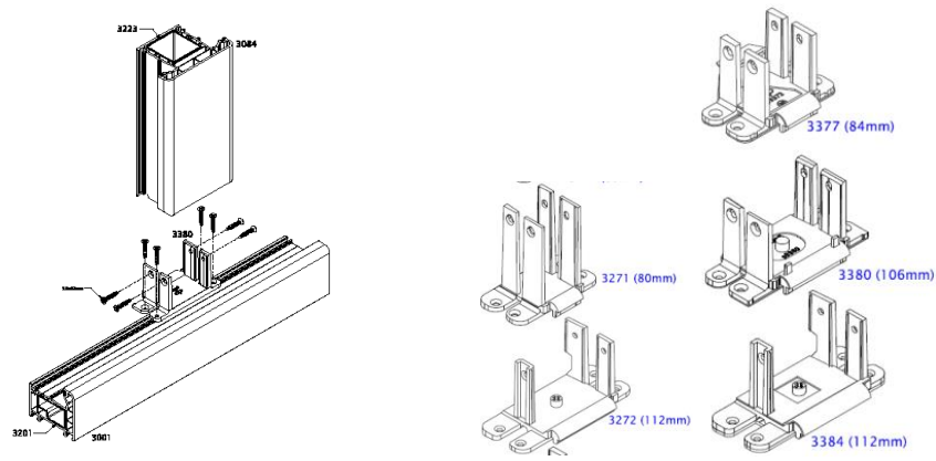
Figuur 2e: Mechanische T-verbinding – type Zamak
