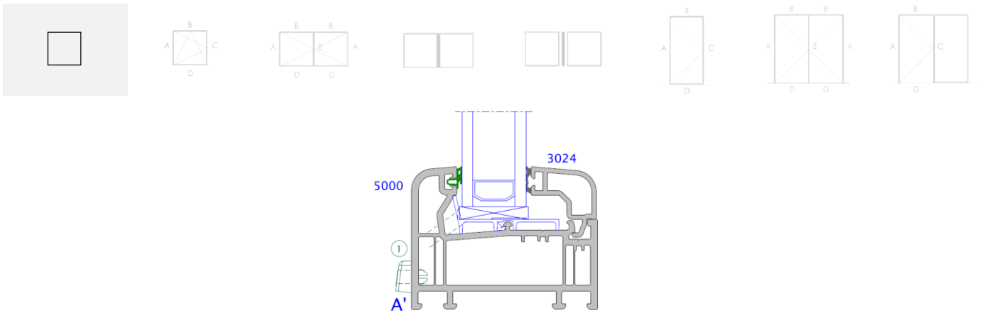
Figuur 7a: Typesnede vast venster
