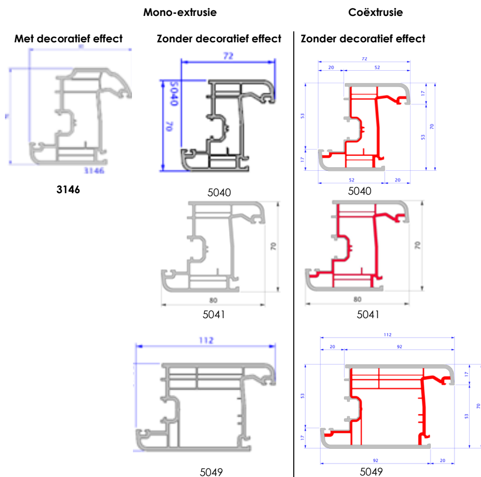
Figuur 2b: Vleugelprofielen
