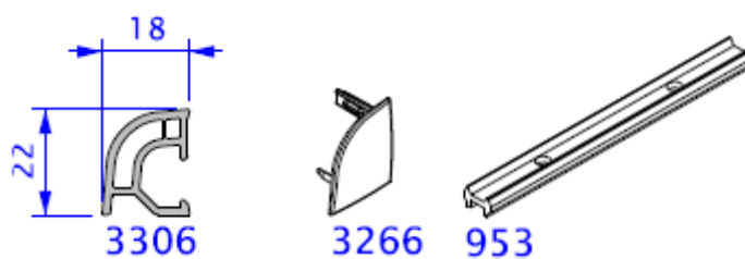
Figuur 5c: Druiplijst
