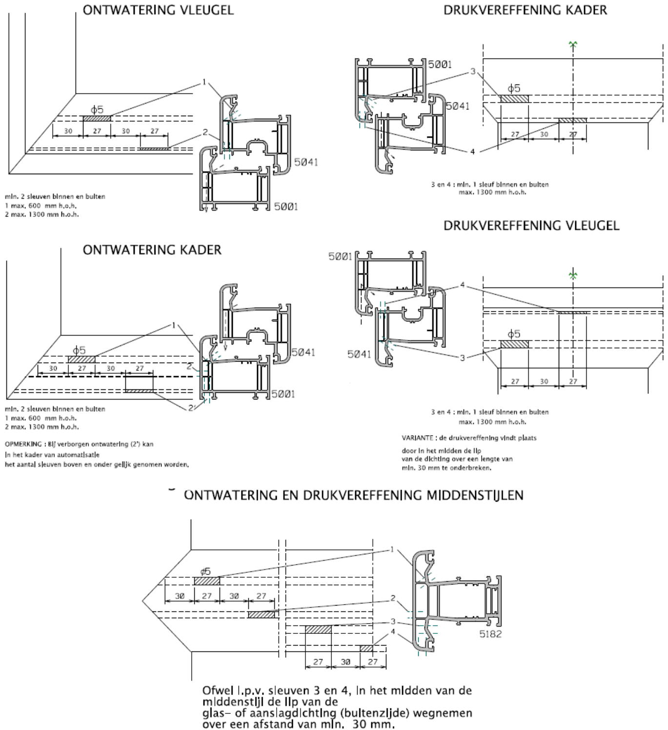
Figuur 8: Ontwatering en drukvereffening kaders en vleugels
