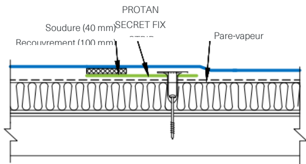
Fig. 14 – Recouvrement des lés (PROTAN SECRET FIX STRIP)
