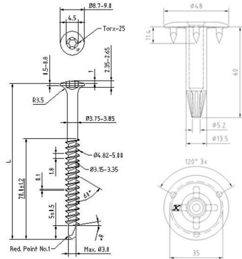
Fig. 2 – Schroef SFS ISOTAK® BS48 + tule SFS ISOTAK® PLUS 48 3-N
