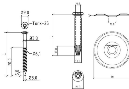
Fig. 8 – Schroef AFAST GUARDIAN® BS61 + plaatje AFAST GUARDIAN® GWSP-80-F4E + tule AFAST GUARDIAN® GWT
