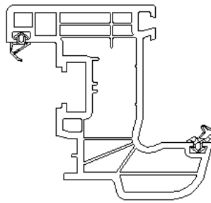
Figure 2b : Profilés d'ouvrant - suite
