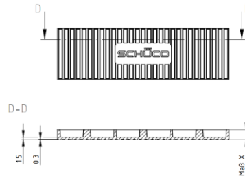
Figure 6.d : Capuchons de drainage
