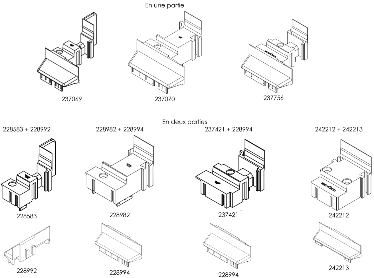
Figure 6.a : Embouts pour maucblairs
