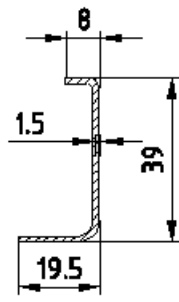
Figure 3 : Profilés de renfort (suite)
