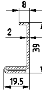
Figure 3 : Profilés de renfort (suite)
