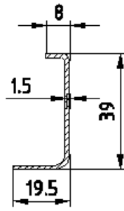
Figuur 3: Versterkingsprofielen (vervolg)
