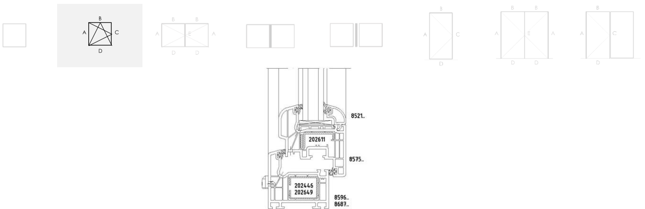
Figuur 7c: Typesnede dubbel opendraaiend venster met makelaar
