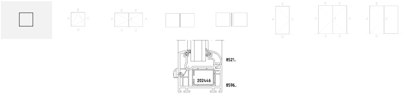
Figuur 7b: Typesnede draai-kip venster
