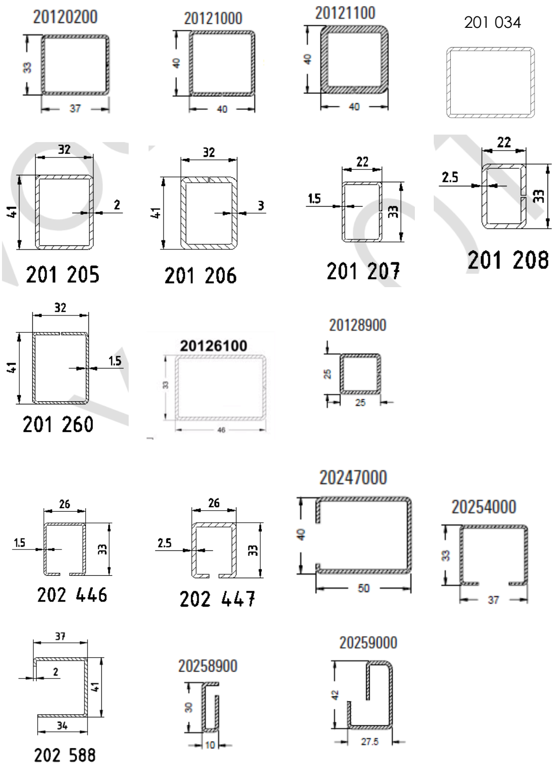
Figuur 3: Versterkingsprofielen
