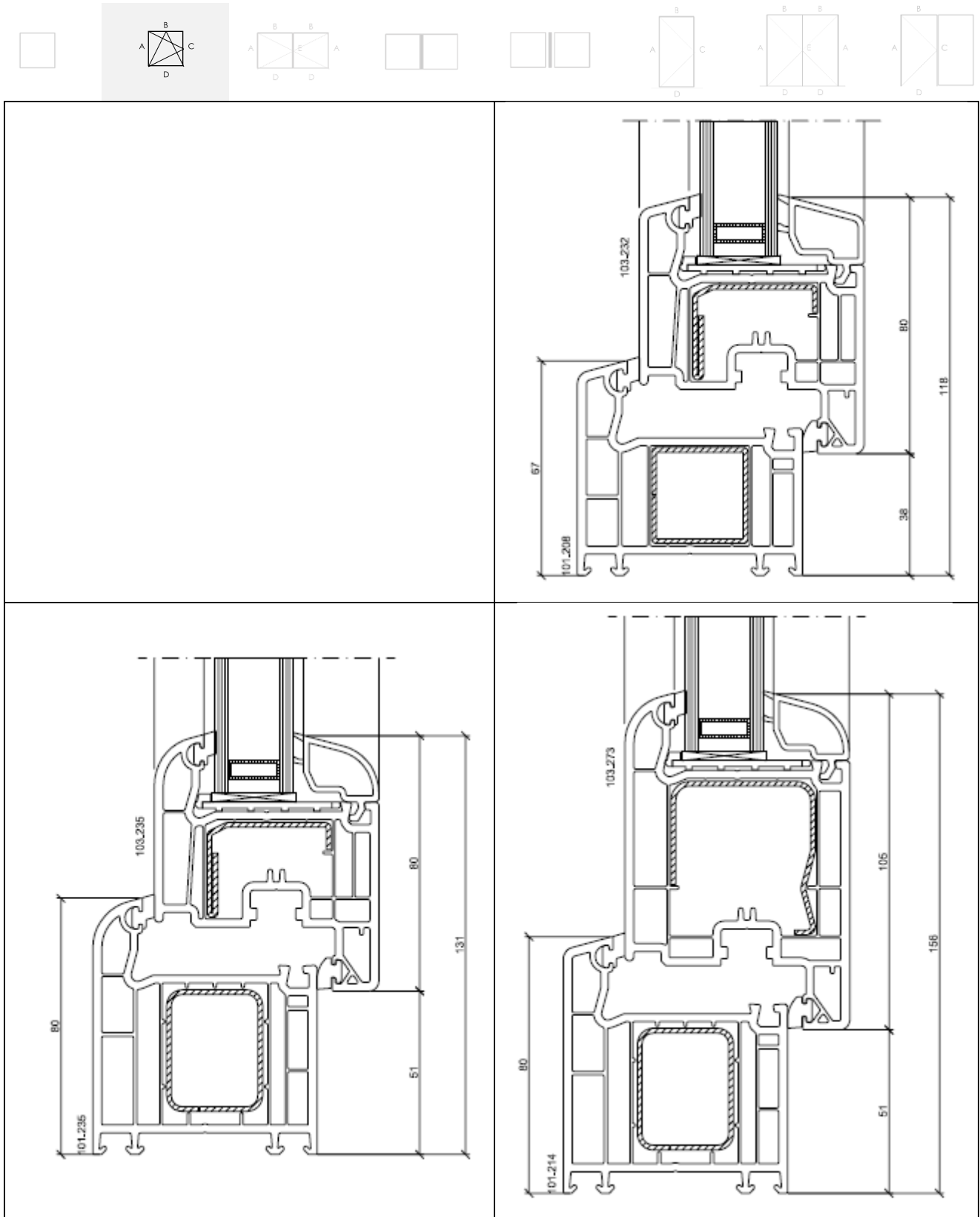
Figure 7b: Coupe-type de fenêtre oscillo-battante
