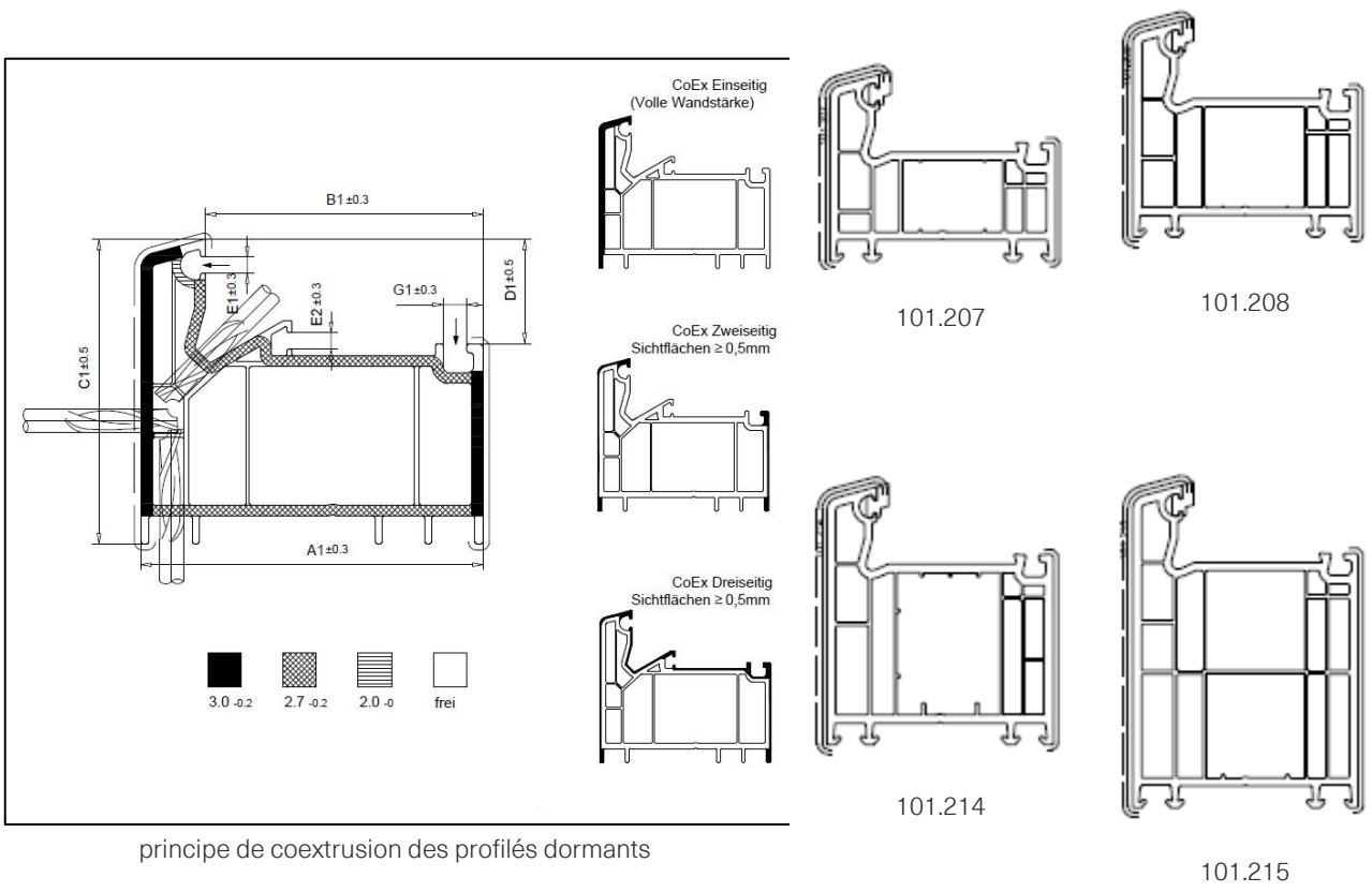
Fig 2a: Profilés dormants
