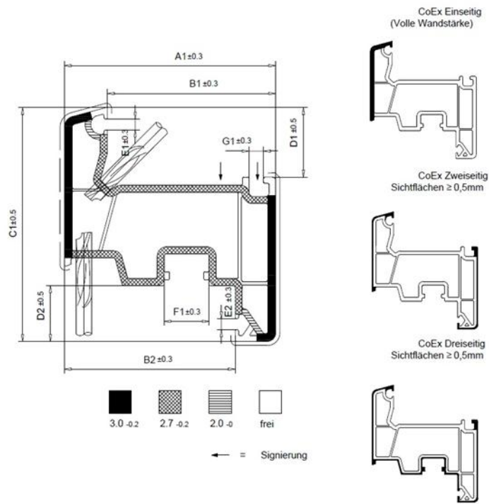
Fig 2b: Profilés d'ouvrant
