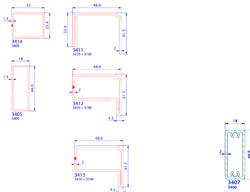
Figure 3: Profilés de renfort métalliques
