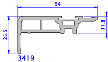
Figure 5.b: Profilés auxiliaires sans fonction de résistance
