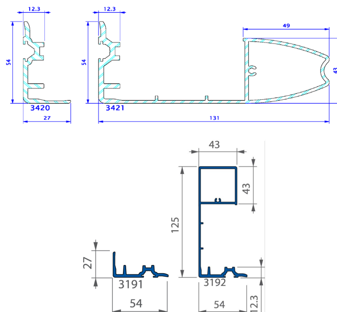
Figure 3: Profilés de renfort métalliques
